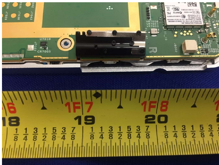
PIFA Antenna
