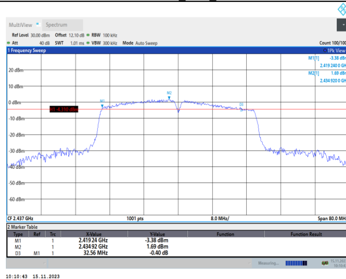
11N40MIMO_Ant2_2437
