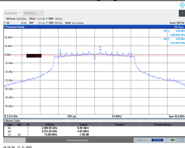
11AC20MIMO_Ant2_2412
