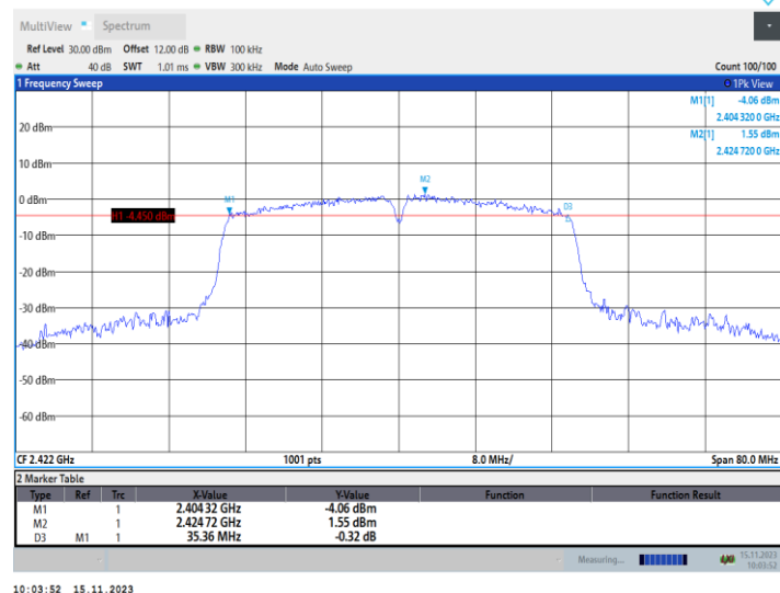
11N40MIMO_Ant2_2422
