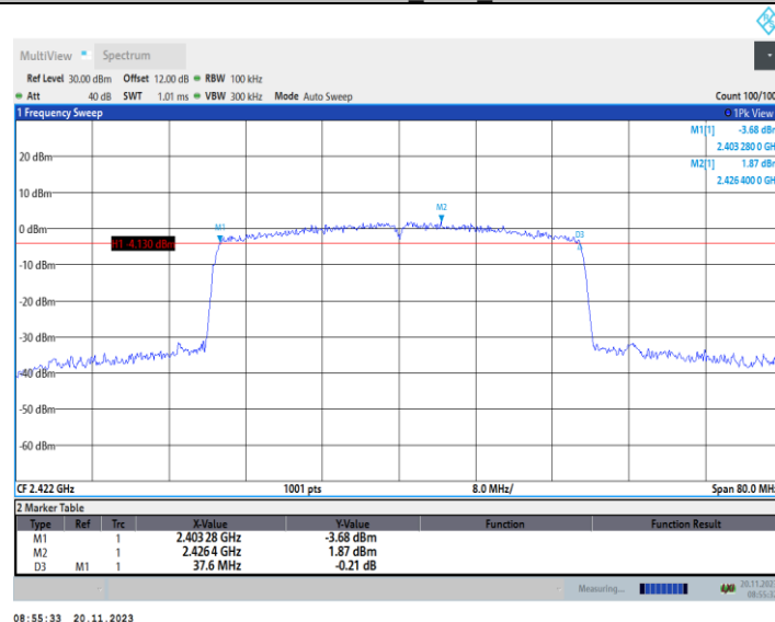
11AX40MIMO Ant2_2422
