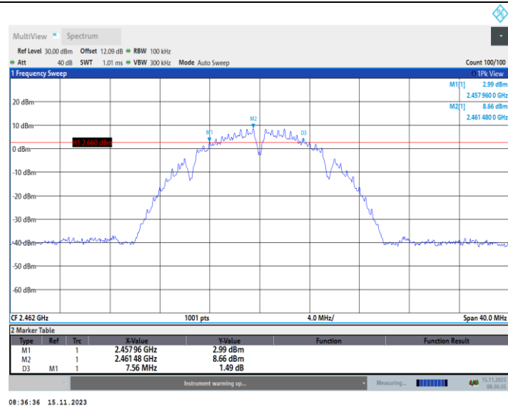
11B_Ant2_2462
