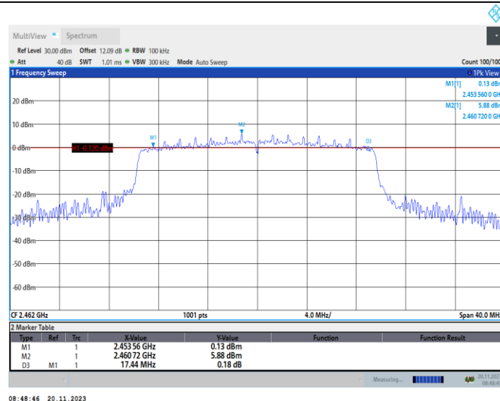
11AX20MIMO Ant2_2462
