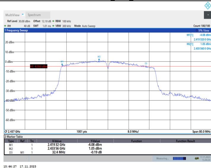
11AC40MIMO Ant2_2437
