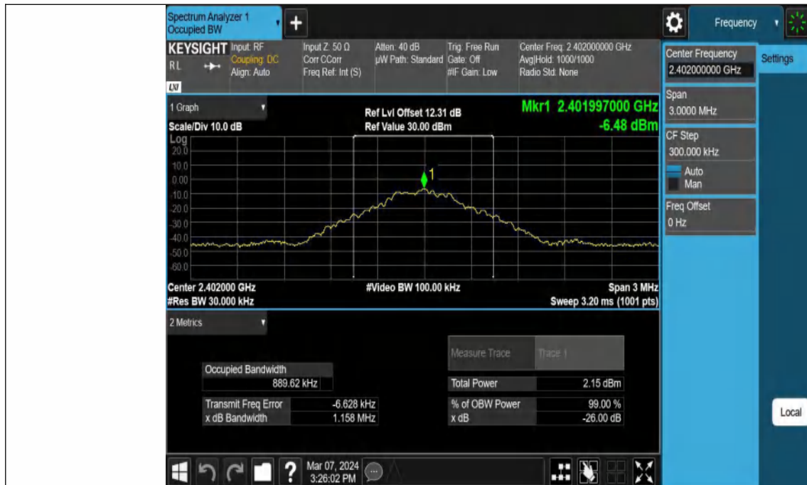
DH5-Ant1-2402
