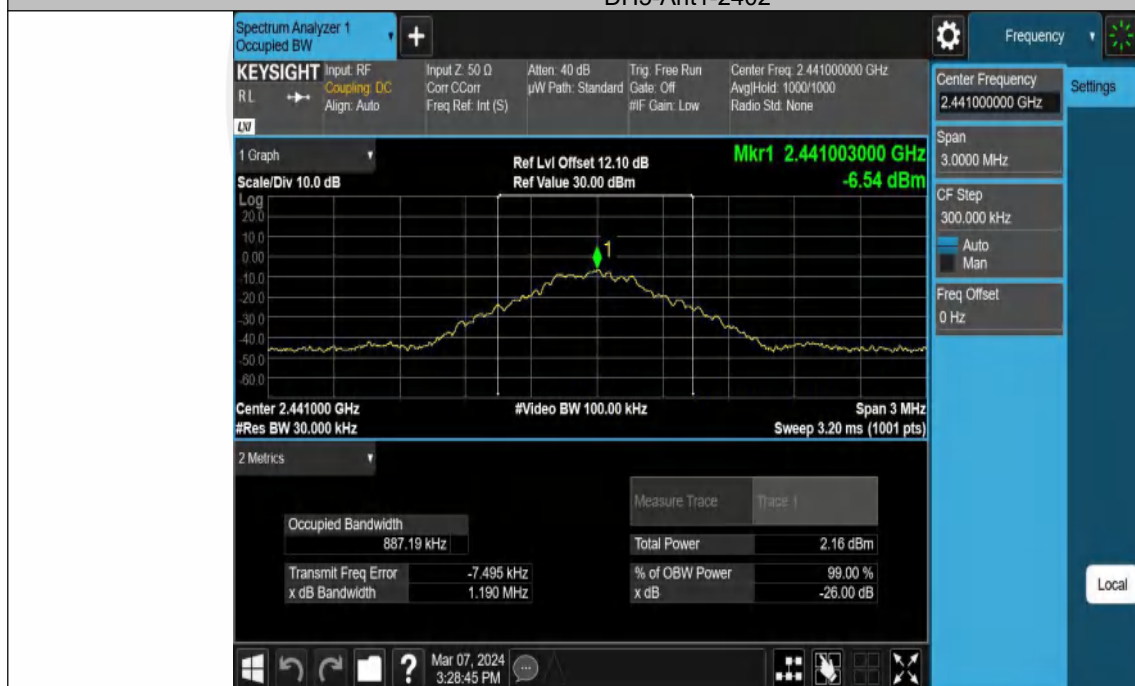
DH5-Ant1-2441
