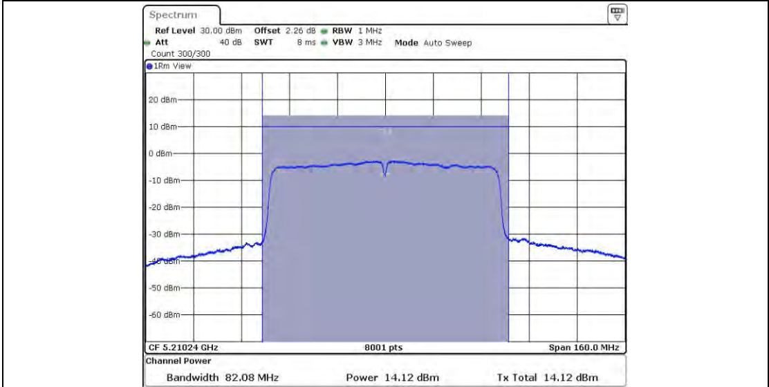
11AC80SISO_Ant1_5210
