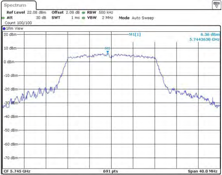
11N20MIMO_Ant2_5745
