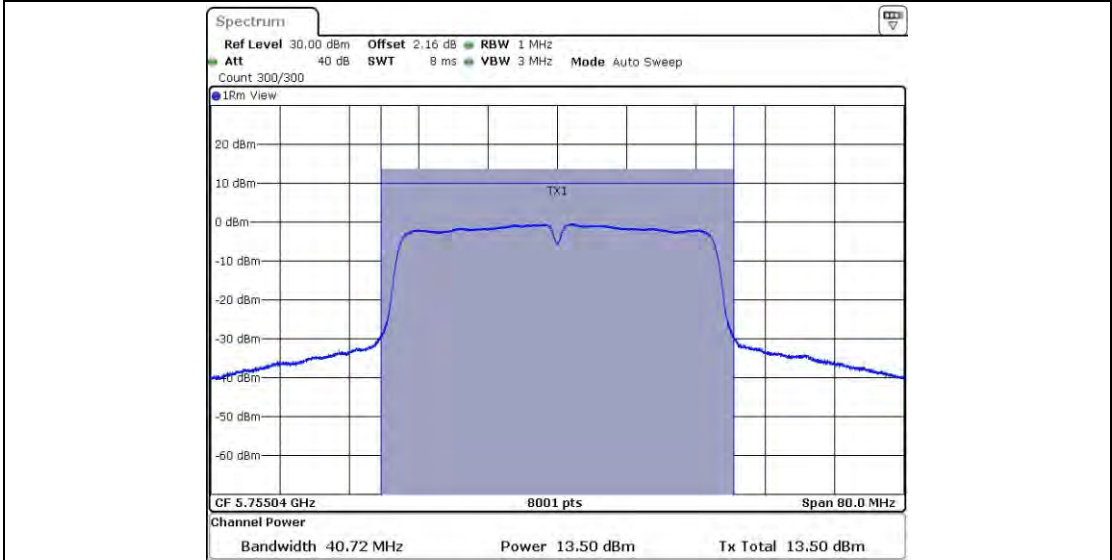
11N40MIMO_Ant1_5755
