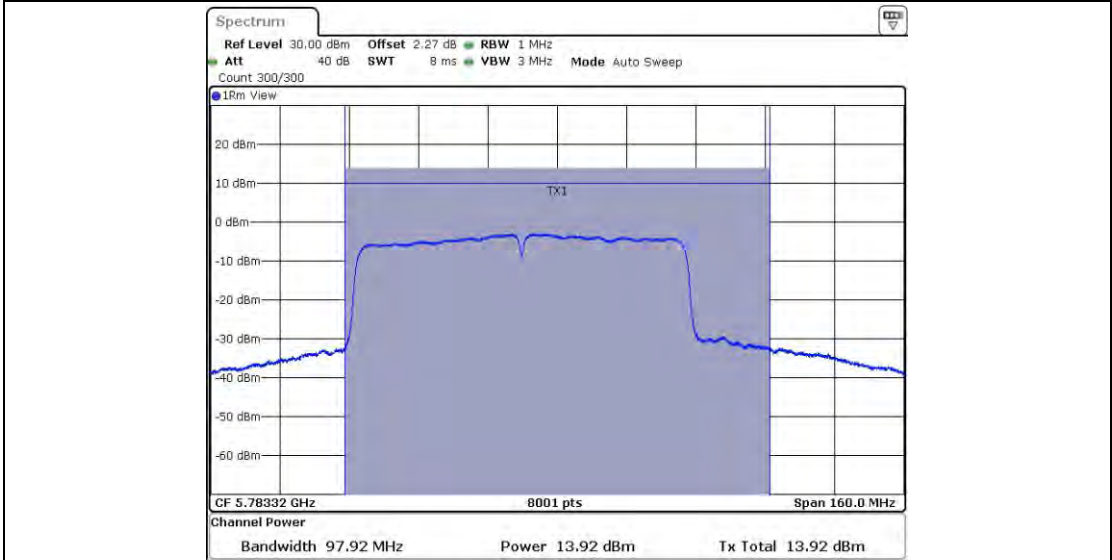
11AC80MIMO_Ant1_5775
