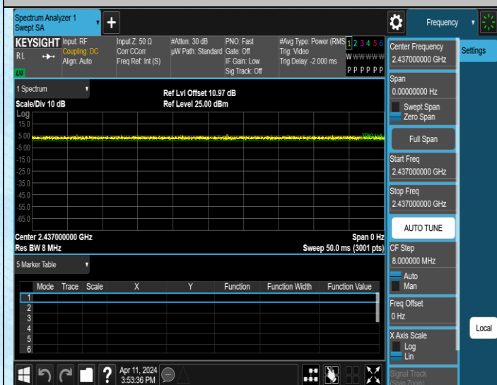
NTNV-11N40MIMO-Ant1-2437
