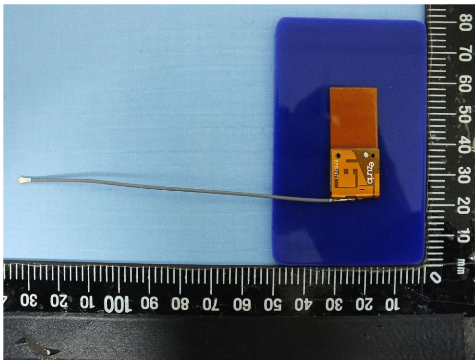
Antenna: FlexPIFA 6E
