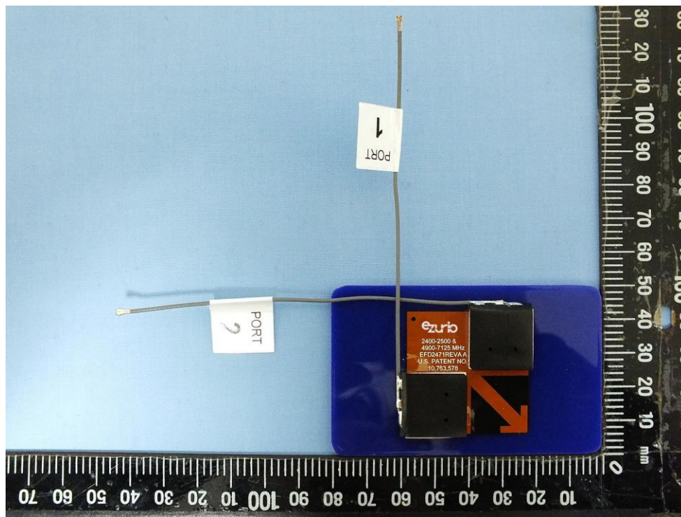
Antenna: FlexMIMO 6E
