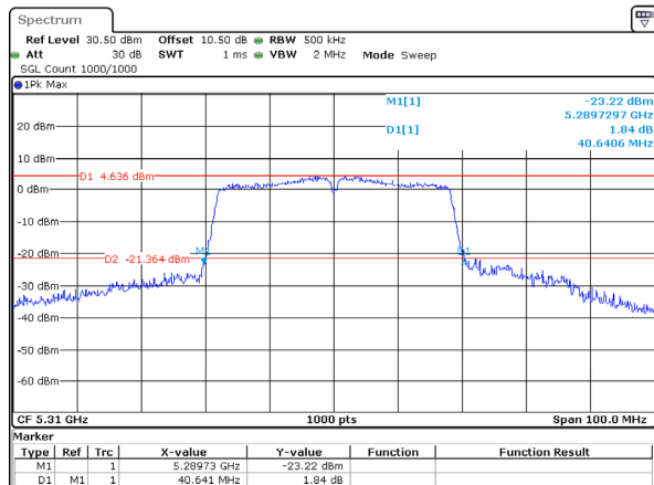
802.11ac40_5310MHz
