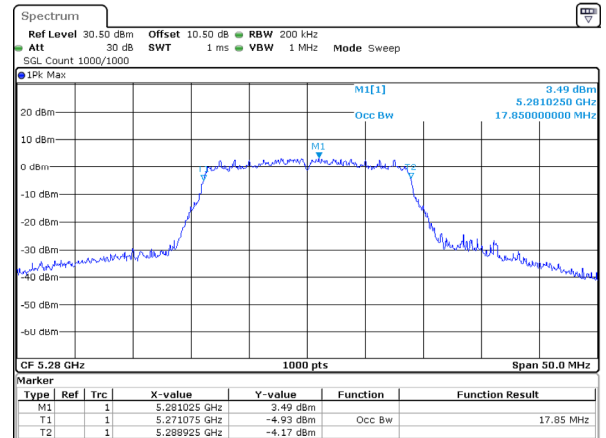
802.11ac20_5280MHz
