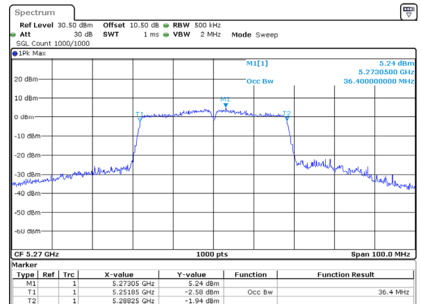
802.11ac40_5270MHz
