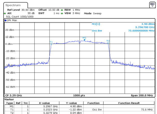
802.11ac80_5290MHz
