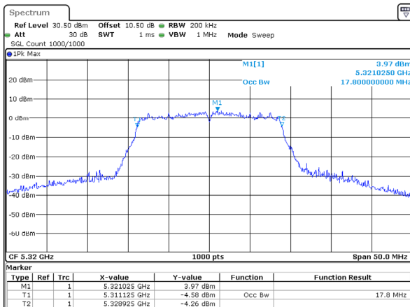
802.11ac20_5320MHz
