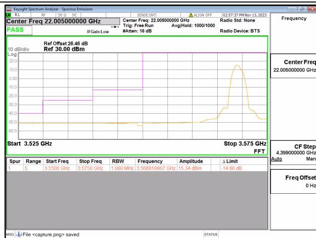
48C / 20+5MHz / Low CH / QPSK / 1#99-1#0
