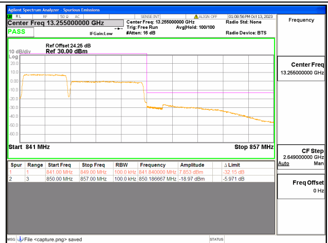
5B / 3+5MHz / High CH / QPSK / 15#0-25#0
