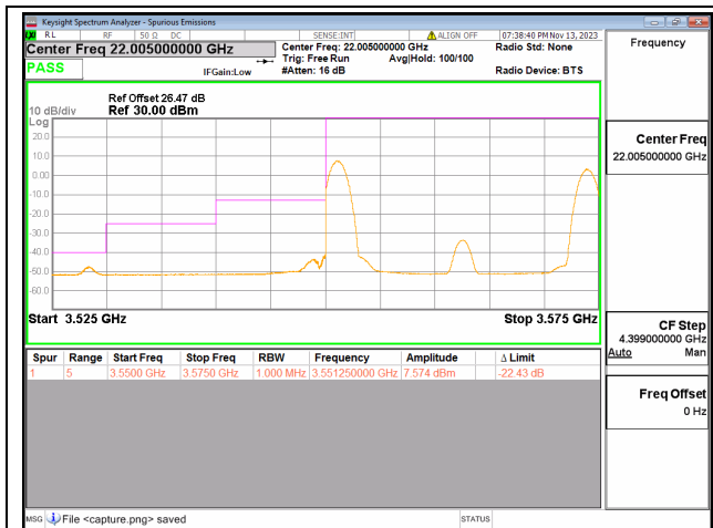
48C / 5+20MHz / Low CH / QPSK / 1#0-1#99
