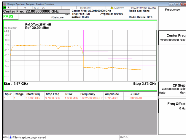
48C / 20+10MHz / High CH / QPSK / 100#0-50#0
