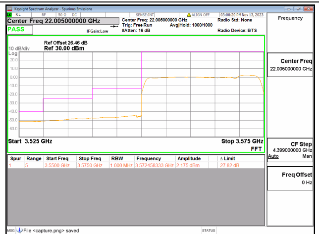
48C / 20+5MHz / Low CH / QPSK / 100#0-25#0
