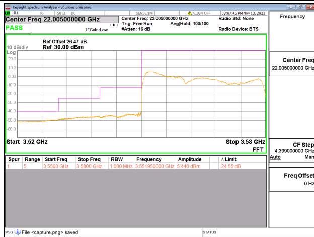
48C / 10+20MHz / Low CH / QPSK / 50#0-100#0
