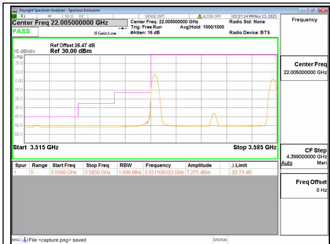
48C / 15+20MHz / Low CH / QPSK / 1#0-1#99
