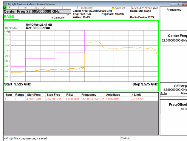
48C / 5+20MHz / Low CH / QPSK / 25#0-100#0
