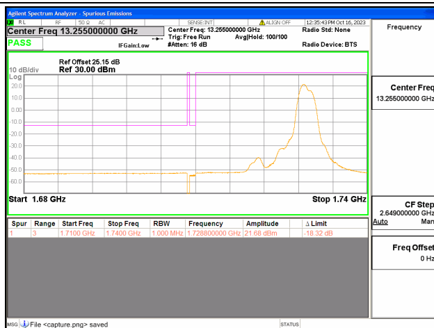
66C / 20+10MHz / Low CH / QPSK / 1#99-1#0
