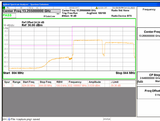
5B / 10+10MHz / Low CH / QPSK / 50#0-50#0
