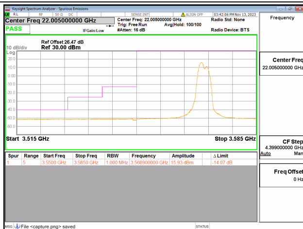
48C / 20+15MHz / Low CH / QPSK / 1#99-1#0
