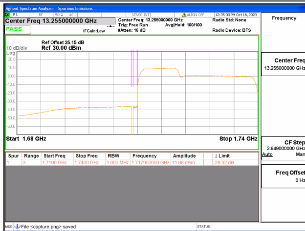
66C / 10+20MHz / Low CH / QPSK / 50#0-100#0
