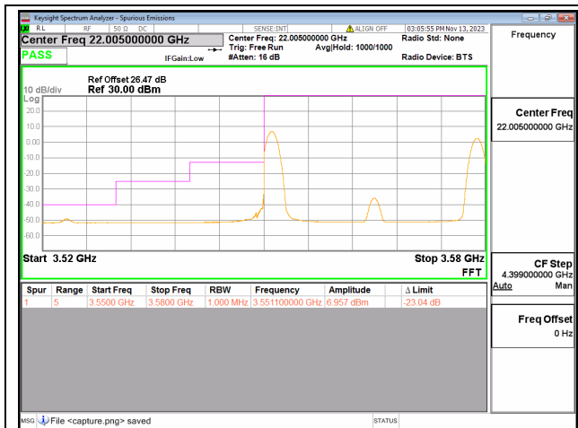
48C / 10+20MHz / Low CH / QPSK / 1#0-1#99
