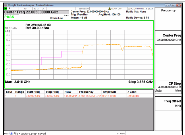
48C / 20+15MHz / Low CH / QPSK / 100#0-75#0
