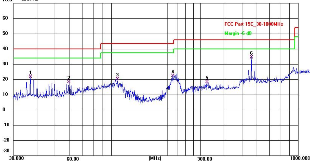
Horizontal dBuV/m
