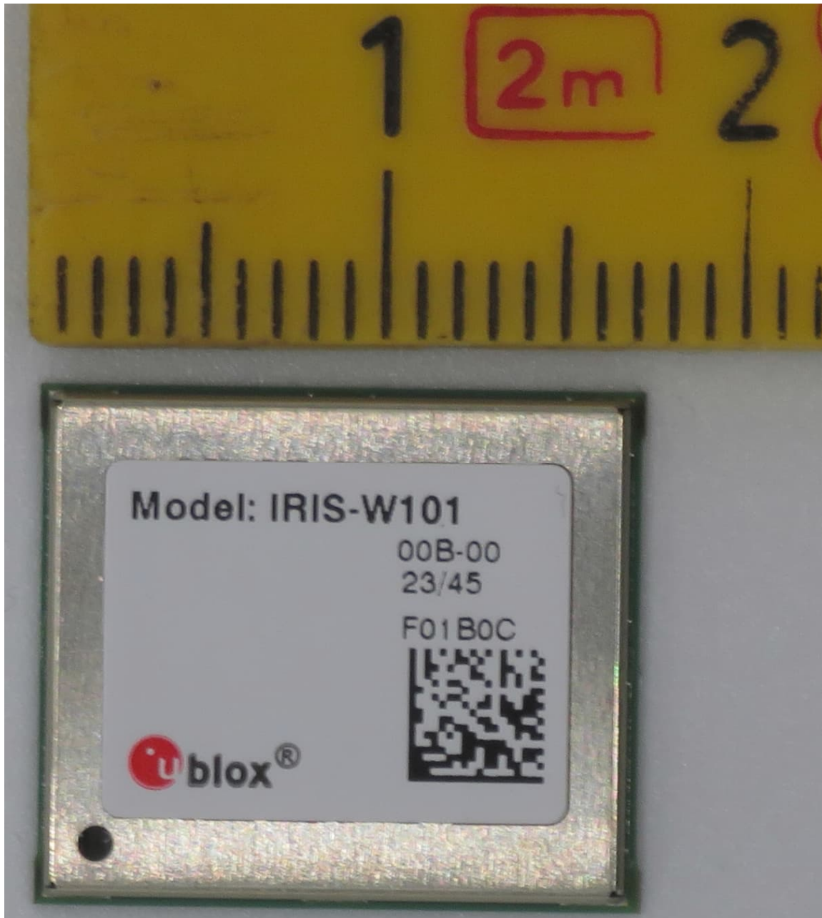
IRIS-W101-00B – top view
