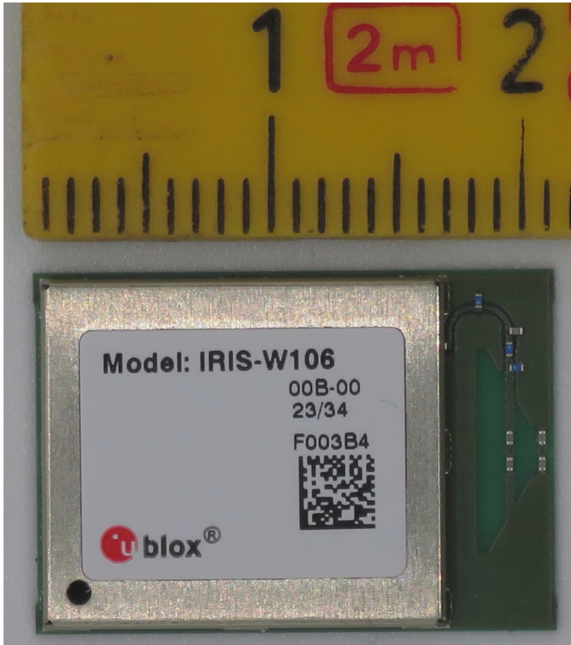
IRIS-W106-00B – top view
