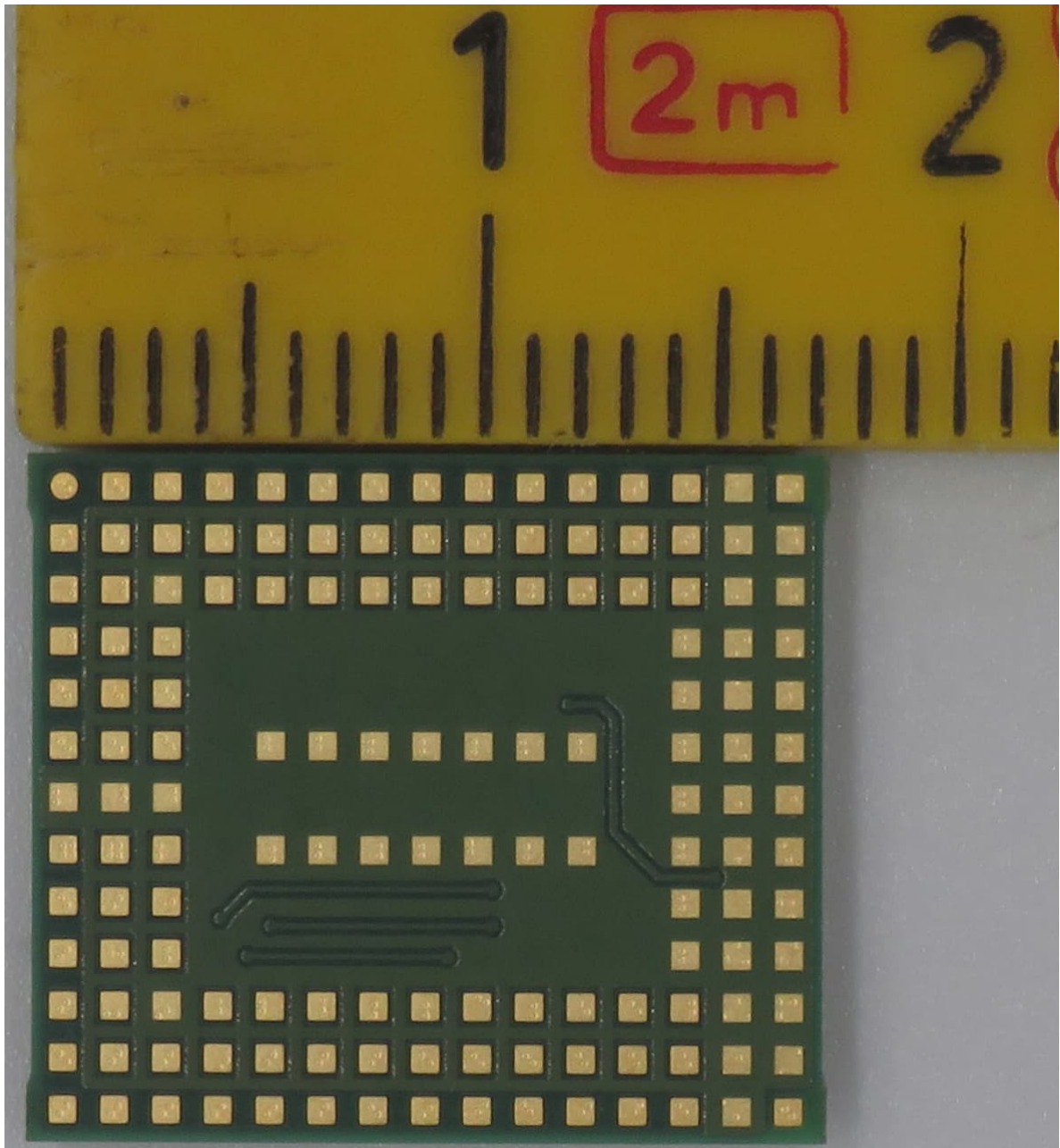
IRIS-W101-00B – bottom view
