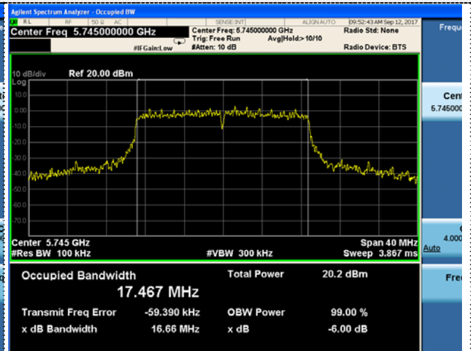
802.11ac(HT20)
