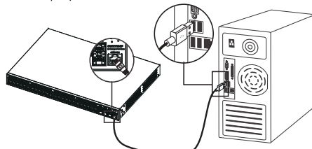
Conecte-se à porta do console (USB)
