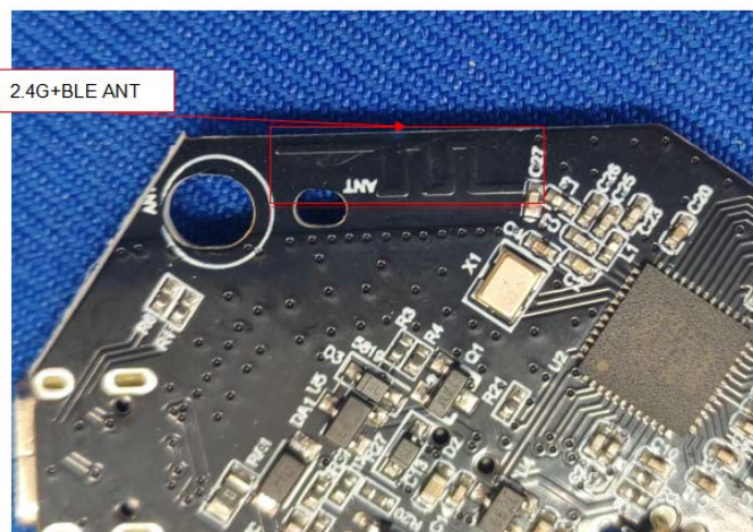
EUT Photo
