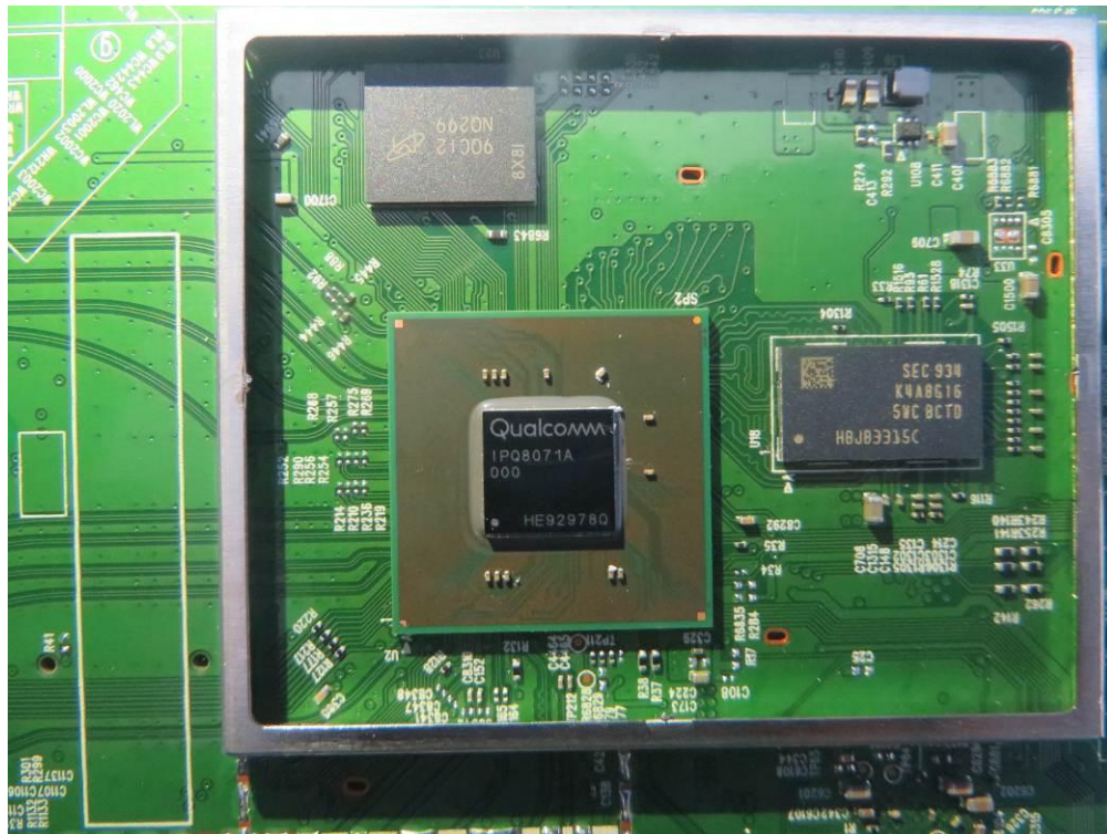
(13) EUT Photo
