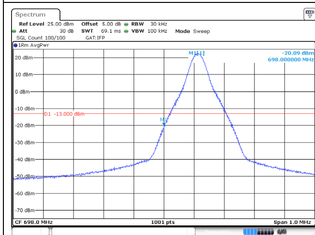
3.75 kHz / BPSK / CH134004 / 1RB0
