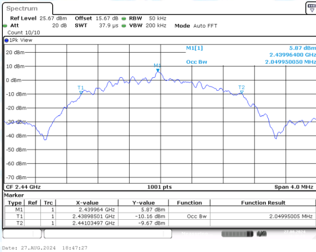
BLE_2M-Ant1-2440
