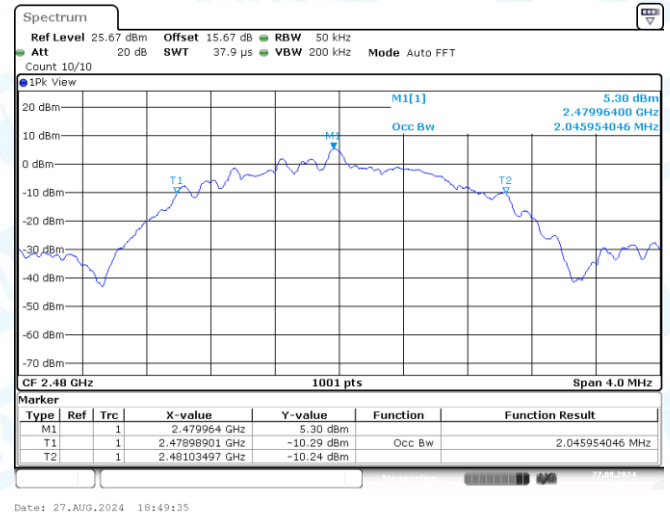
BLE_2M-Ant1-2480
