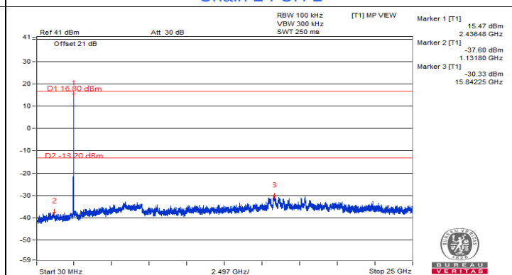
Chain 2 : CH 6
