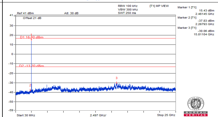
Chain 2 : CH 11
