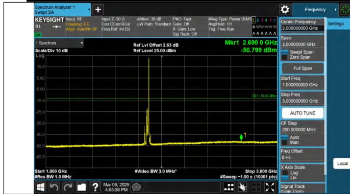
Band2-20MHz-QPSK-18900-1RB#99-1000~3000-PASS
