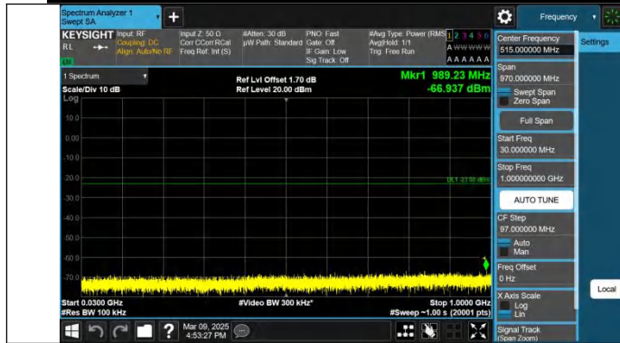
Band2-20MHz-QPSK-18700-1RB#0-30~1000-PASS
