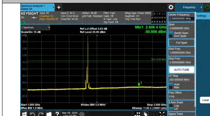
Band2-20MHz-QPSK-18700-1RB#99-1000~3000-PASS
