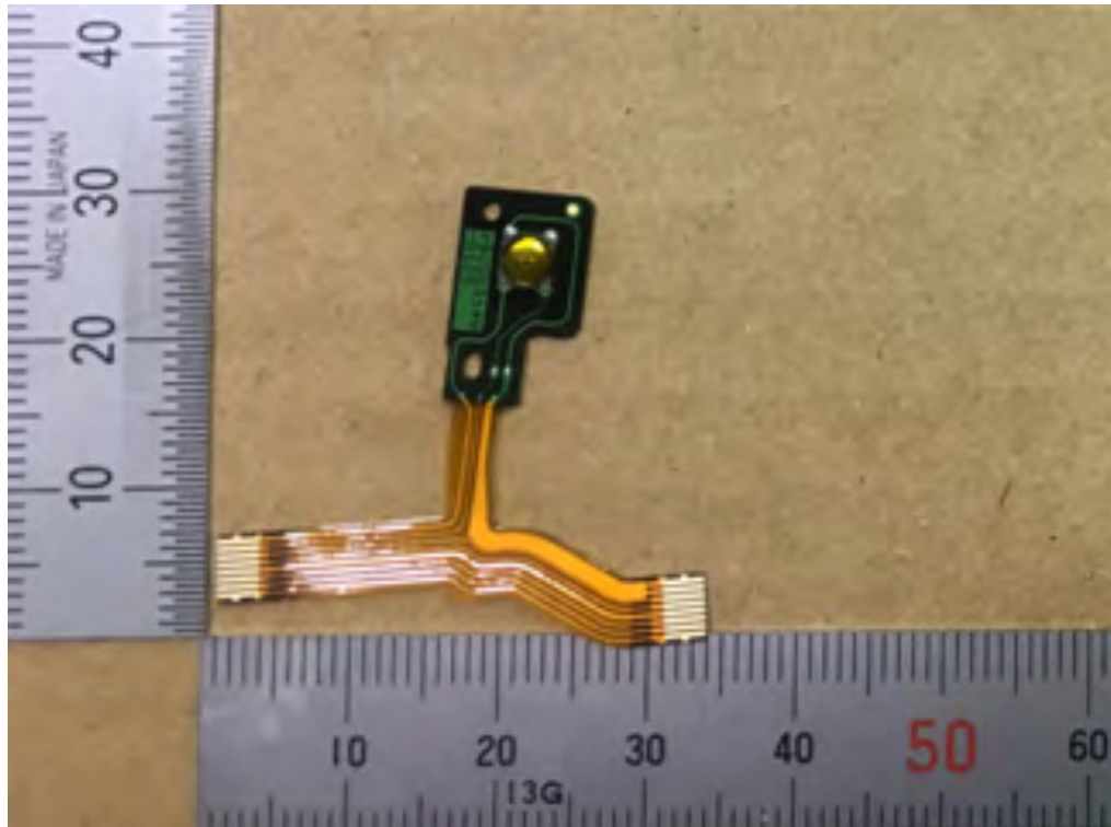
FPC Q_A
