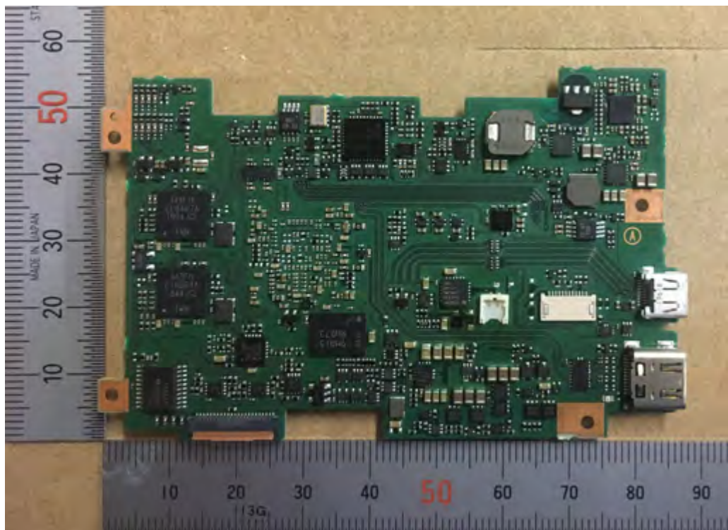
PWB MAIN_B
