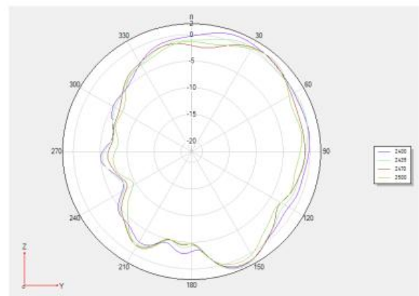
Phi 90 2D图
