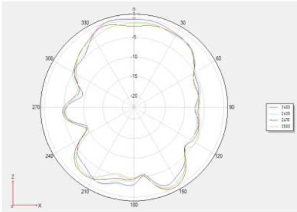
Phi 0 2D图
