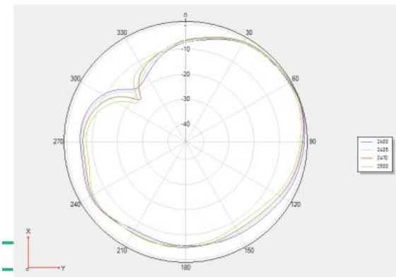
Theta 90 2D图
