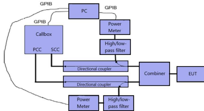
(d) Appendix A – Test Setup Photo 3
