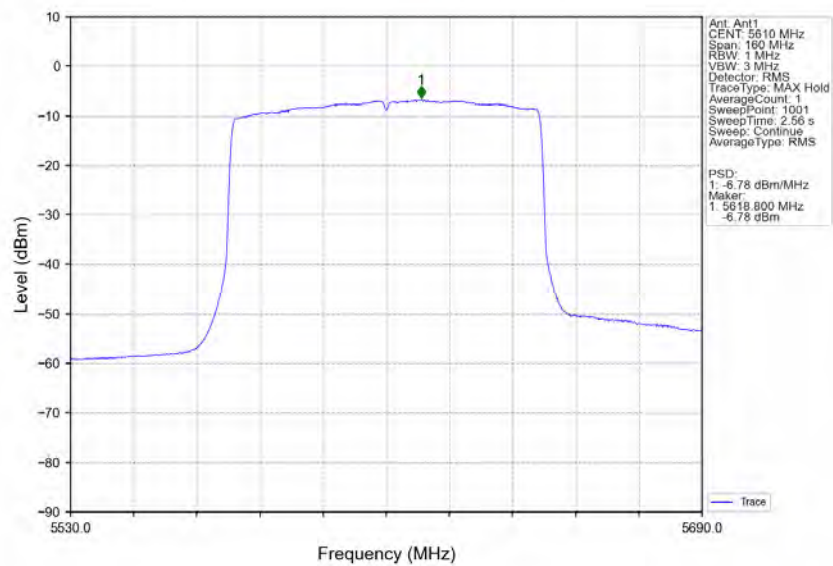
802.11ax(HEW80) HCH 5610MHz RU996 Left Ant1 NTN
