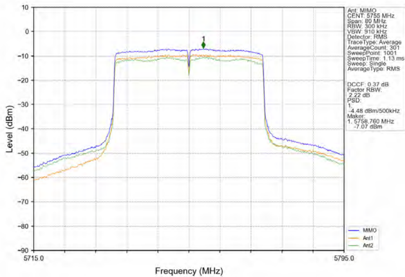
802.11ax(HEW40) LCH 5755MHz RU484 Left MIMO NTN
