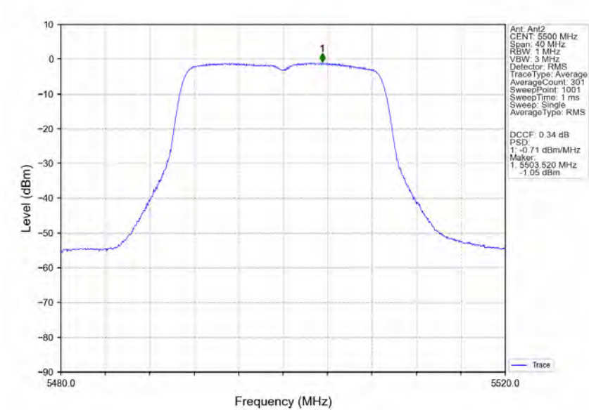
802.11ac(VHT20) LCH_5500MHz_Ant2_NTNV
