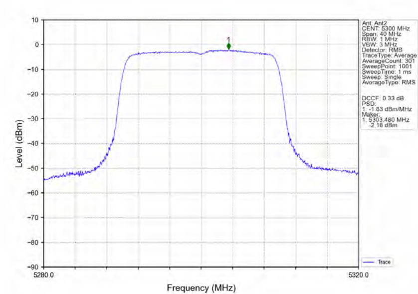
802.11ax(HEW20) MCH_5300MHz RU242 Left Ant2 NTN
