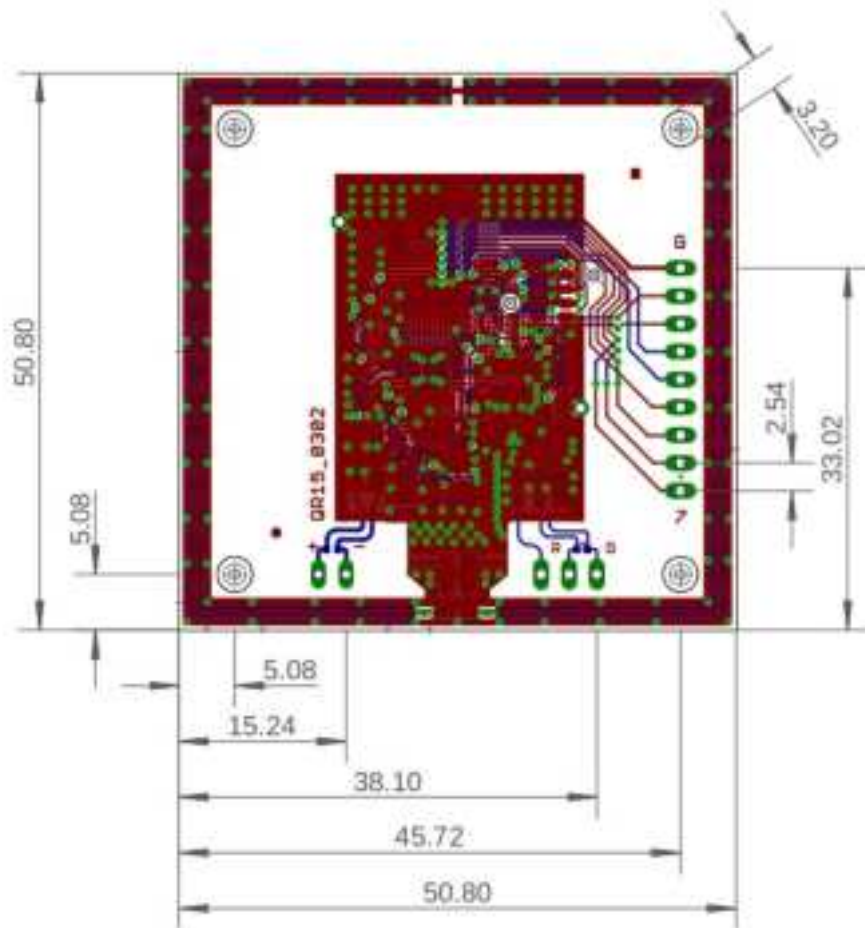
Fig. 3: Mechanical Dimensions QR15 v2
