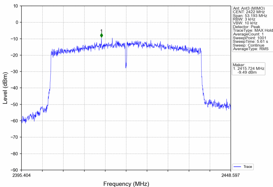
802.11ax(HEW40)_LCH_2422MHz_RU484_Left_Ant3 (MIMO)_NTNV
