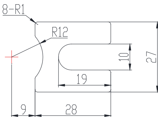
尺寸图
