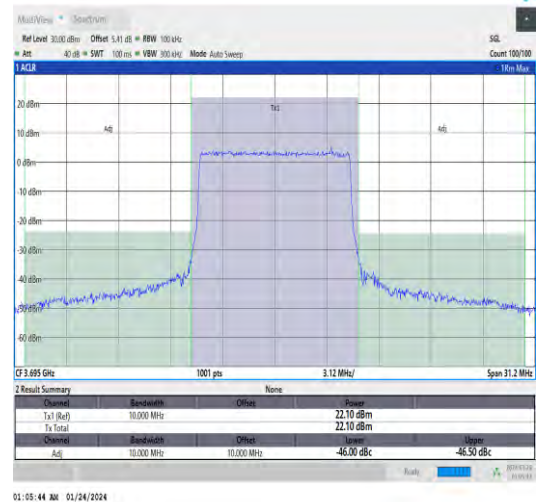
Band48-10MHz-QPSK-56690-50RB#0-PASS
