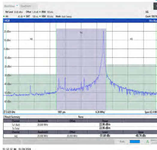
Band48-20MHz-QPSK-55990-1RB#99-PASS
