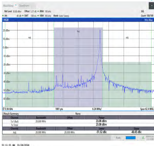
Band48-20MHz-QPSK-55340-1RB#99-PASS
