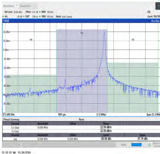
Band48-10MHz-QPSK-56690-1RB#49-PASS
