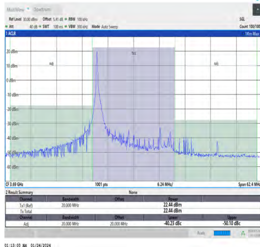
Band48-20MHz-QPSK-56640-1RB#0-PASS
