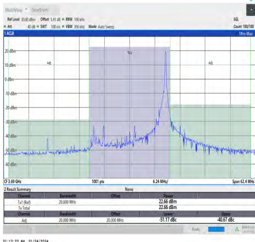
Band48-20MHz-QPSK-56640-1RB#99-PASS
