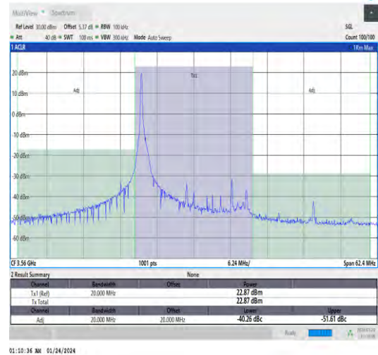
Band48-20MHz-QPSK-55340-1RB#0-PASS
