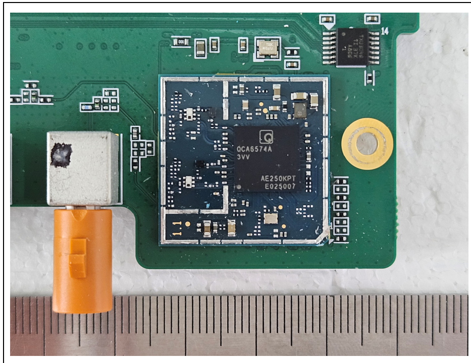
<BT, WLAN Module>
