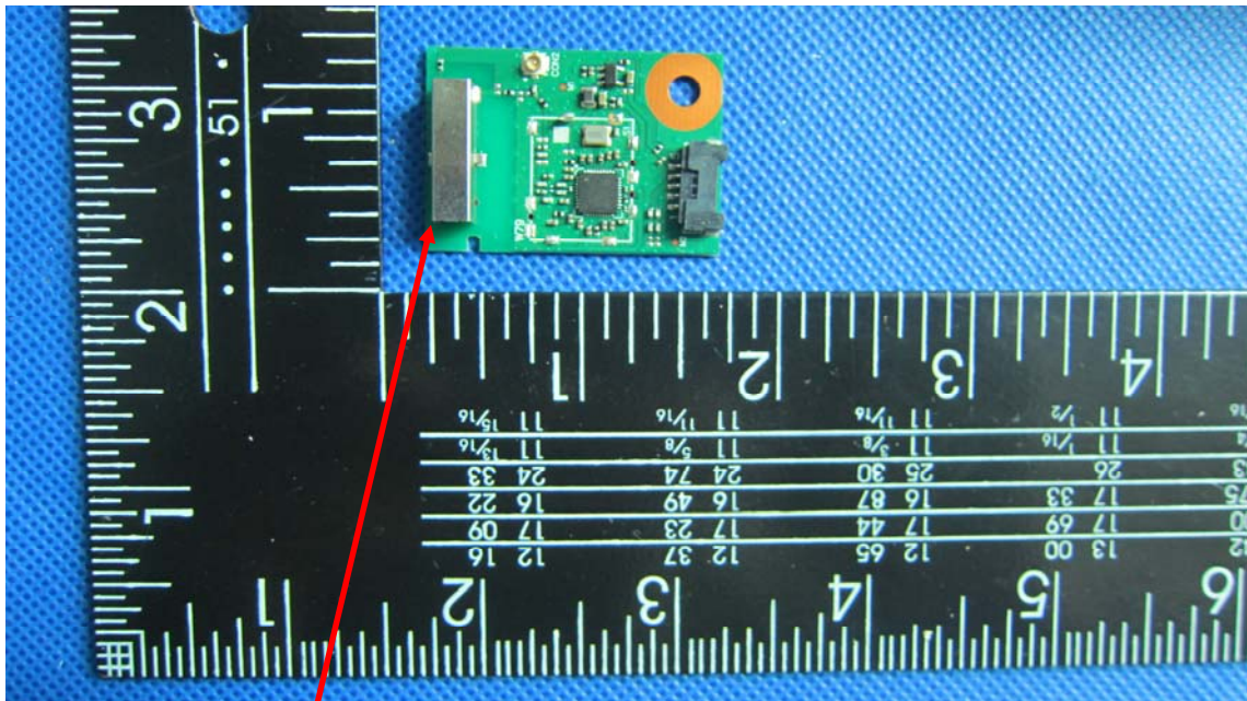
PIFA Antenna 0
