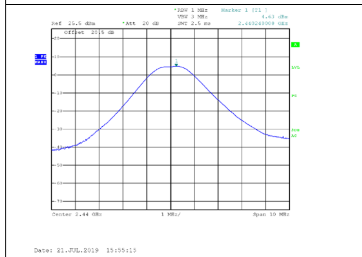
Figure 18. 2440.0 MHz, BLE
