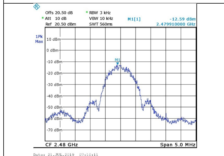
Figure 28. 2480.0 MHz, BLE
