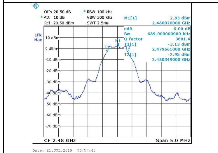
Figure 14. 2480.0 MHz, BLE
