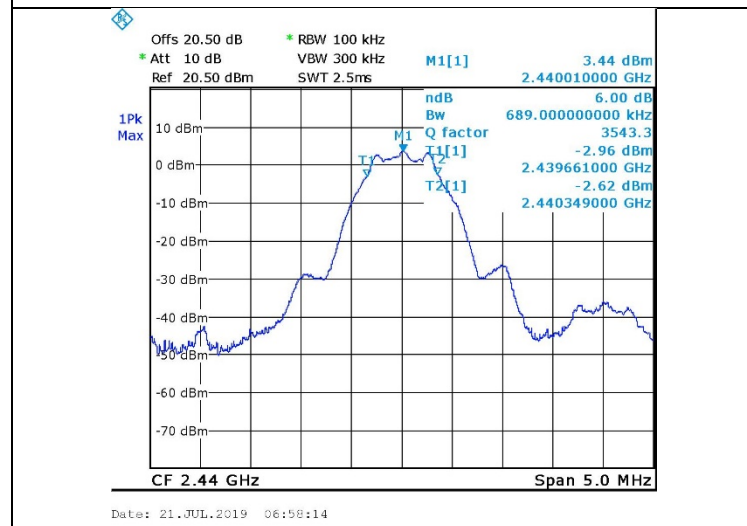
Figure 13. 2440.0 MHz, BLE
