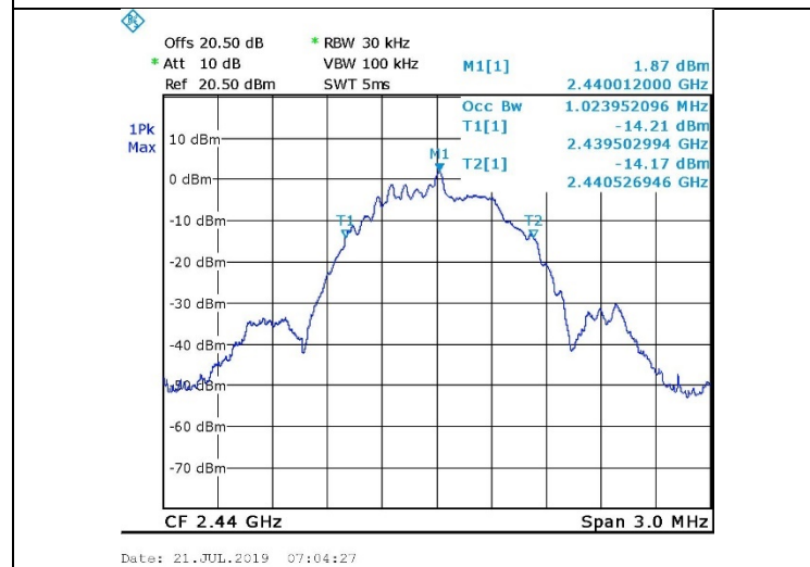
Figure 32. 2440.0 MHz, BLE
