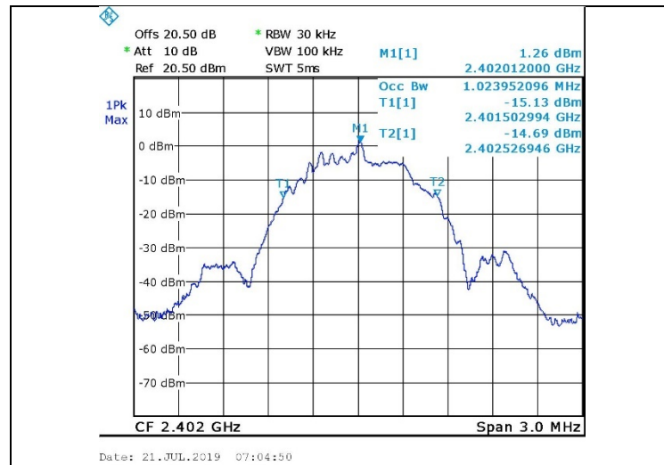
Figure 31. 2402.0 MHz, BLE
