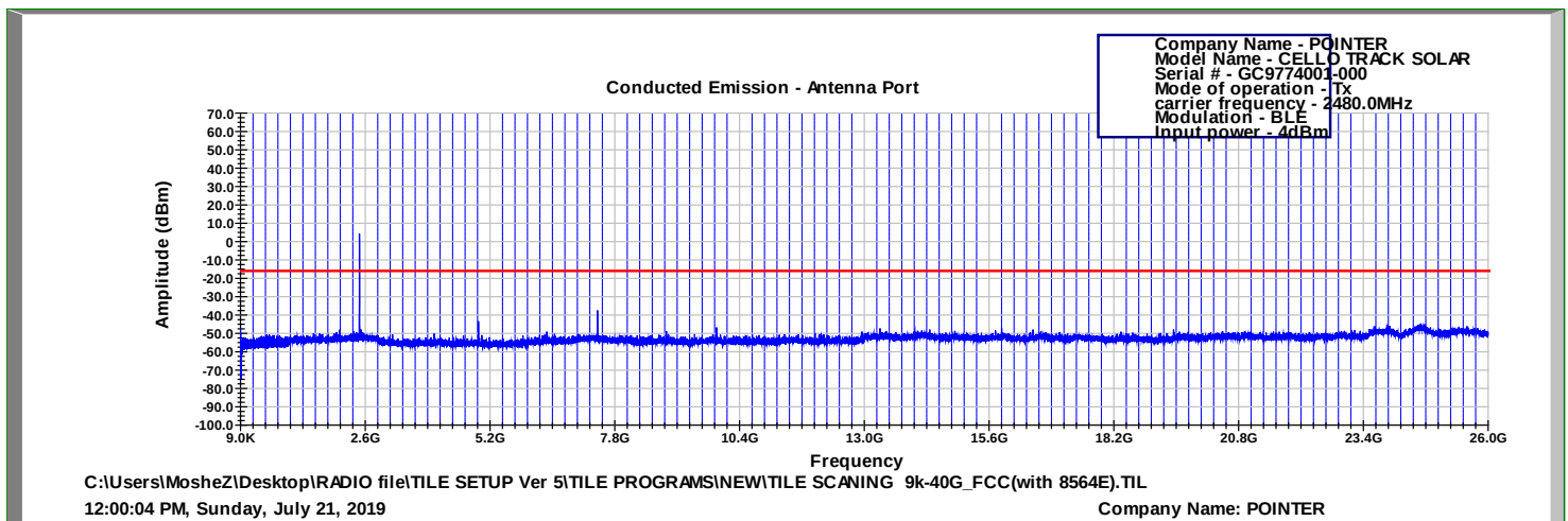
Figure 37 2480.0 MHz, BLE
