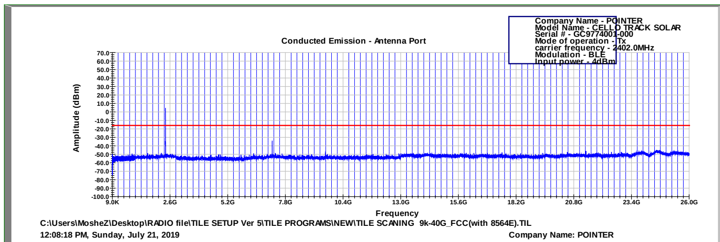
Figure 35 2402.0 MHz, BLE
