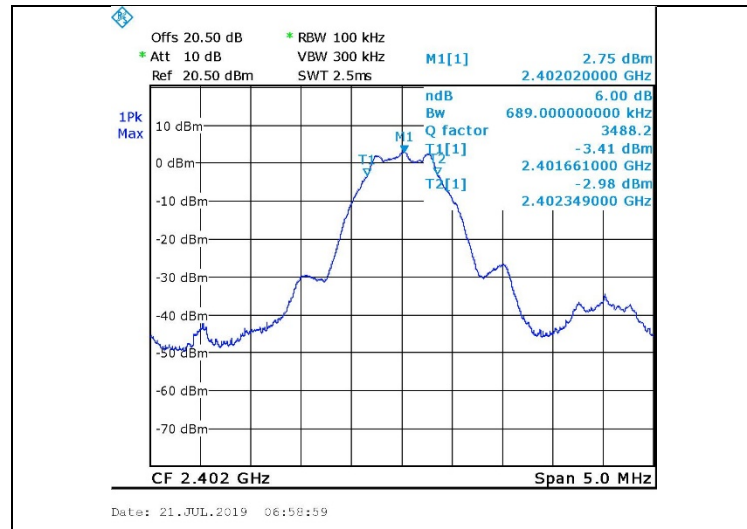
Figure 12. 2402.0 MHz, BLE
