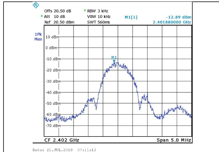
Figure 26. 2402.0 MHz, BLE
