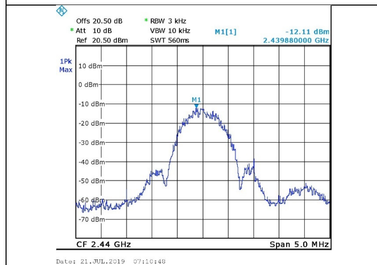
Figure 27. 2440.0 MHz, BLE
