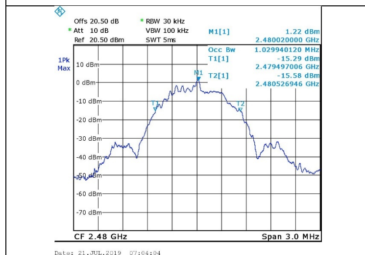
Figure 33. 2480.0 MHz, BLE
