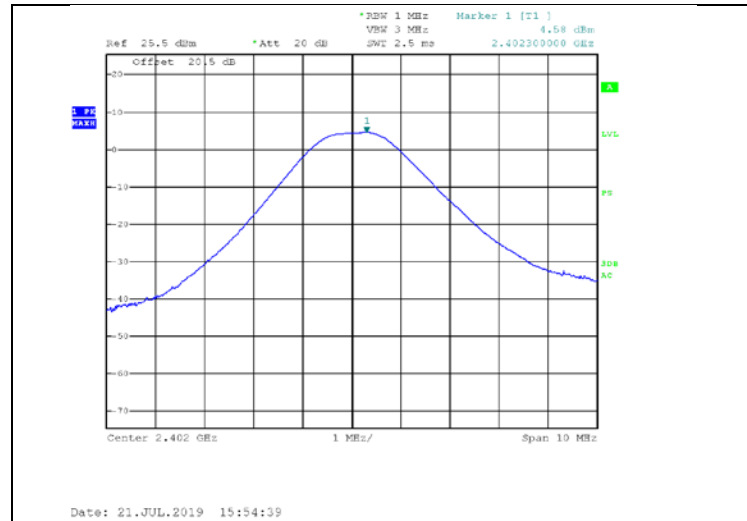
Figure 17. 2402.0 MHz, BLE
