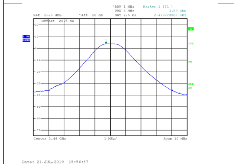
Figure 19. 2480.0 MHz, BLE
