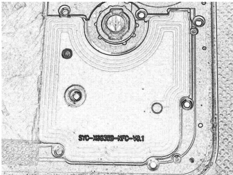
NFC Antenna
