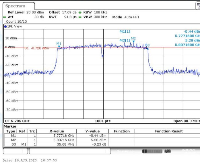
11AC40MIMO_Ant2_5795
