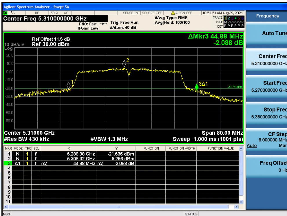
11N40MIMO-Ant3-5310
