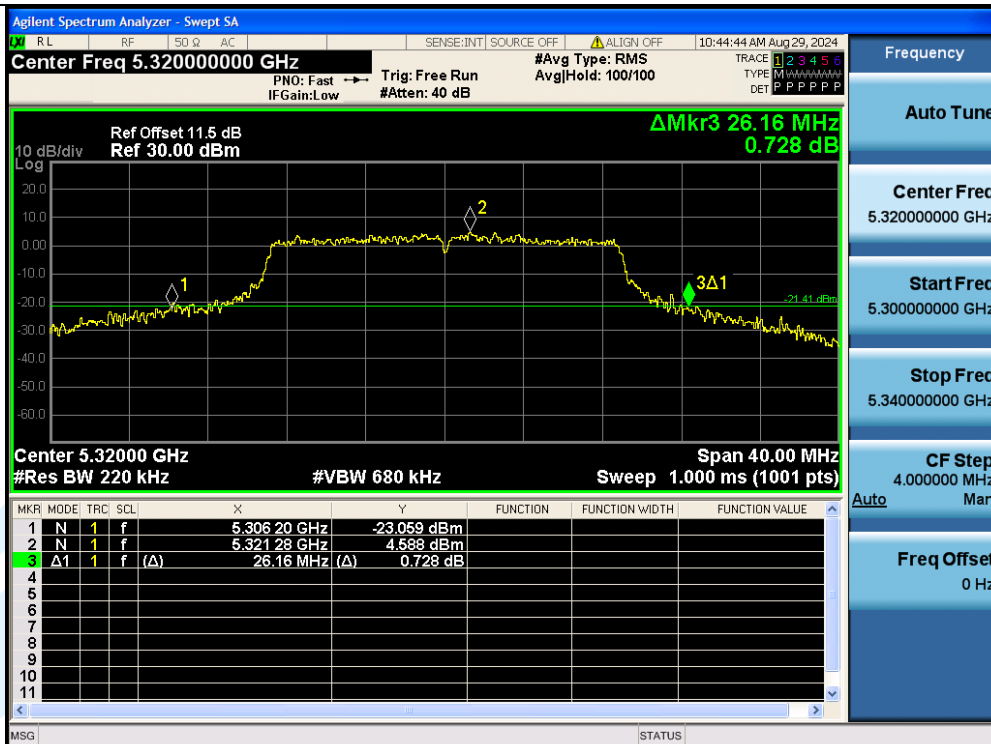
11N20MIMO-Ant3-5320
