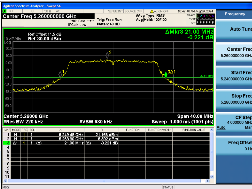
11N20MIMO-Ant3-5260
