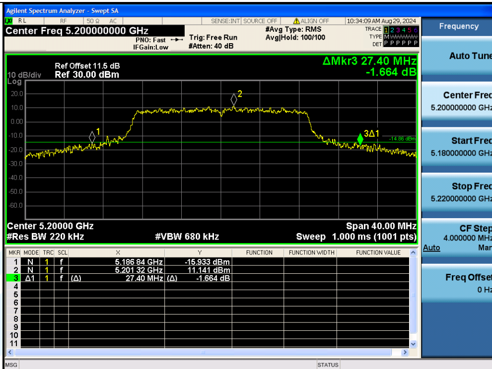
11N20MIMO-Ant3-5200
