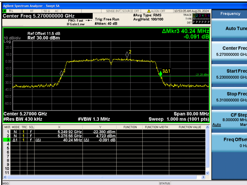
11N40MIMO-Ant3-5270
