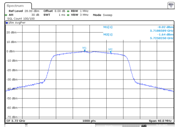
802.11n20_5720MHz_Chain 0
