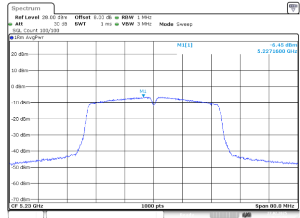
802.11n40_5230MHz_Chain 1
