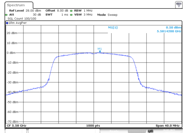
802.11n20_5580MHz_Chain 0
