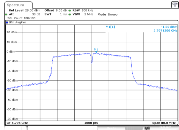
802.11n40_5795MHz_Chain 1
