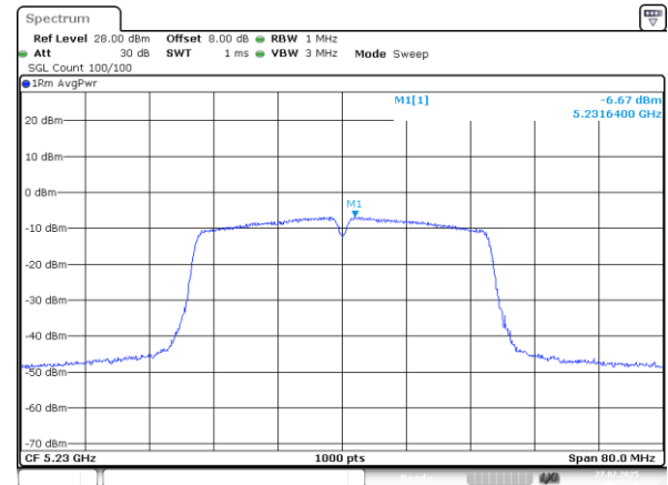
802.11n40_5230MHz_Chain 0
