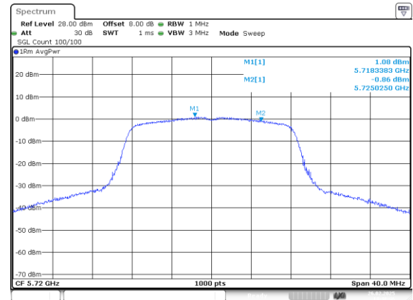
802.11a_5720MHz_Chain 1
