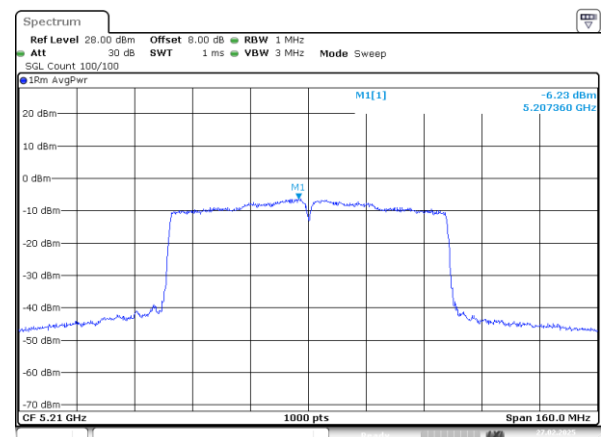
802.11ac80_5210MHz_Chain 1
