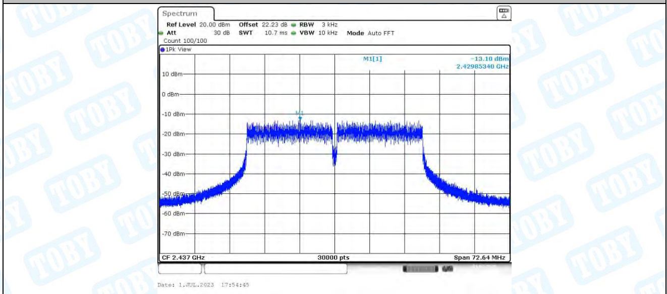
11N40MIMO_Ant2_2437
