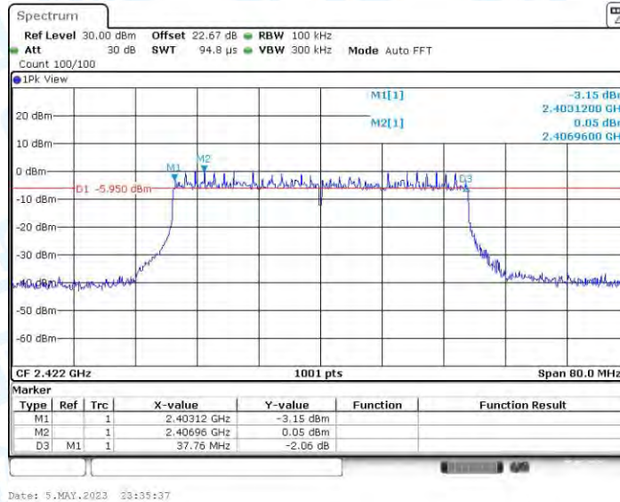
11AX40MIMO_Ant3_2422
