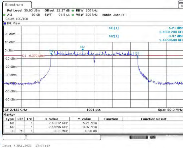
11AX40MIMO_Ant3_2452
