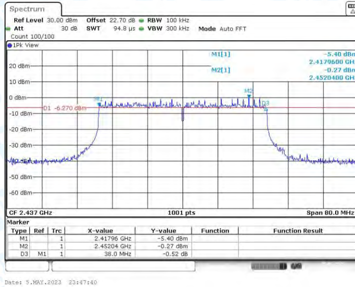
11AX40MIMO_Ant4_2437
