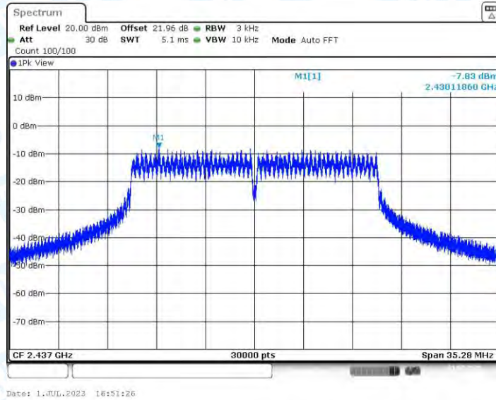
11N20MIMO_Ant4_2437
