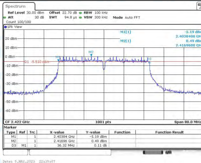
11N40MIMO_Ant4_2422
