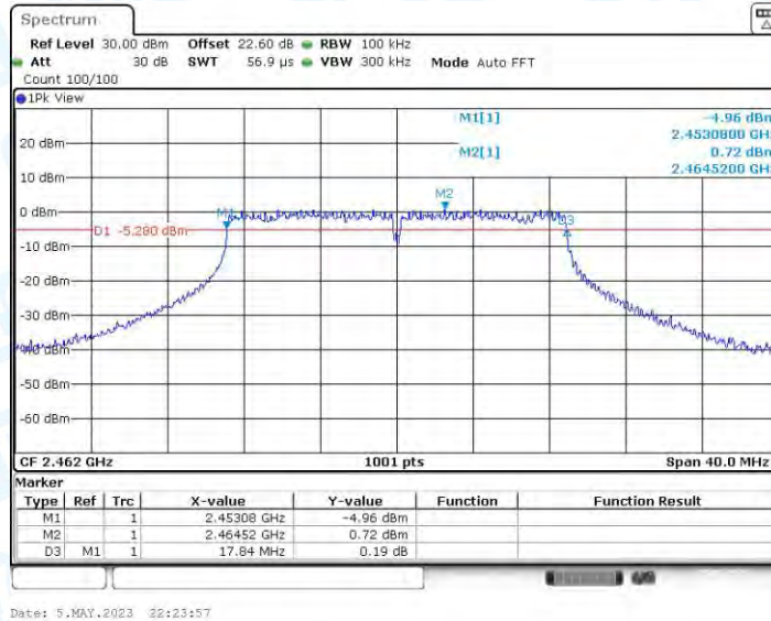
11N20MIMO_Ant4_2462
