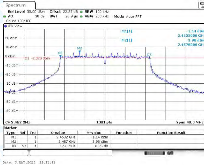
11N20MIMO_Ant3_2462
