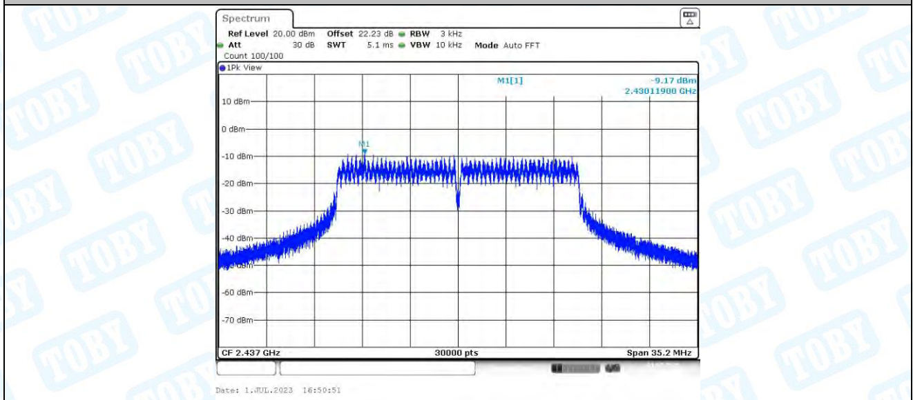
11N20MIMO_Ant2_2437
