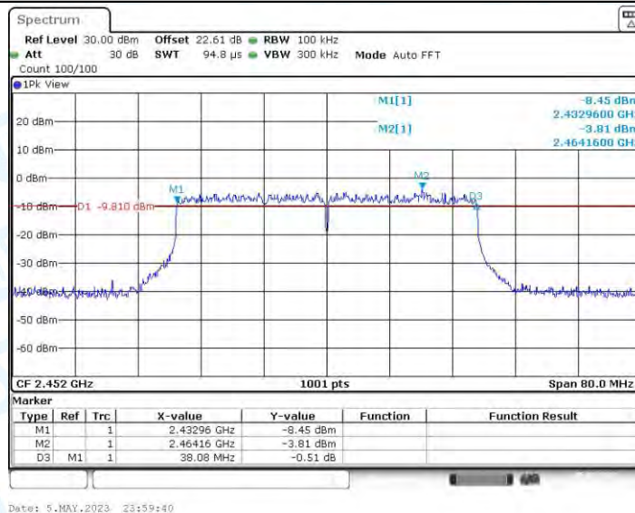
11AX40MIMO_Ant4_2452
