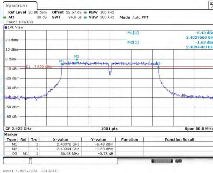
11N40MIMO_Ant3_2422
