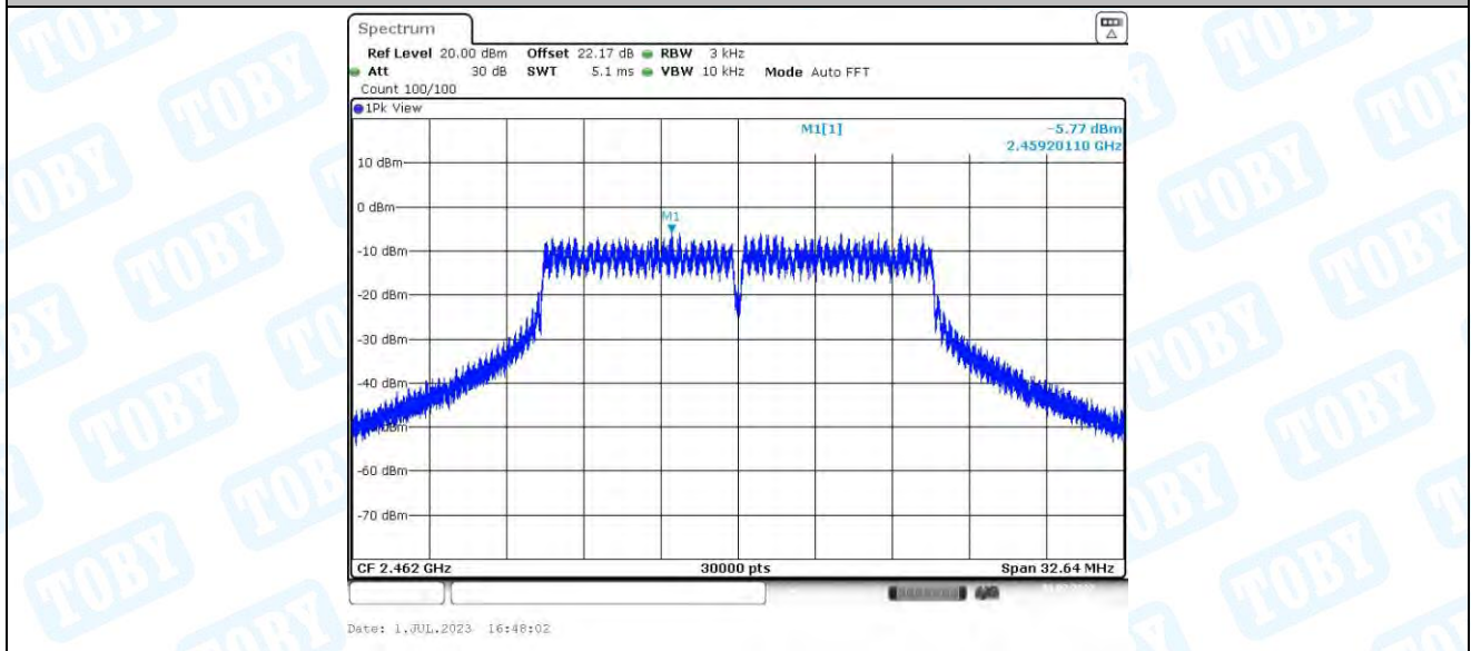
11G_Ant2_2462
