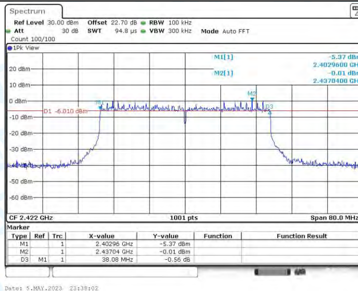
11AX40MIMO_Ant4_2422
