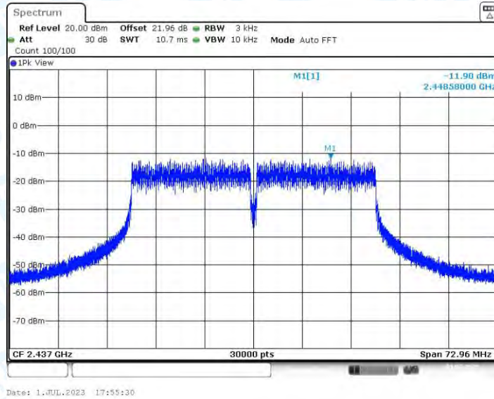
11N40MIMO_Ant4_2437
