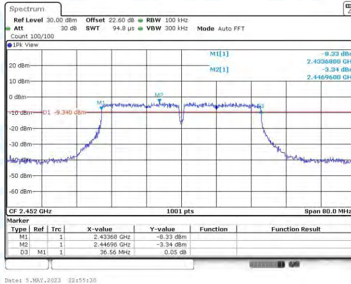
11N40MIMO_Ant4_2452
