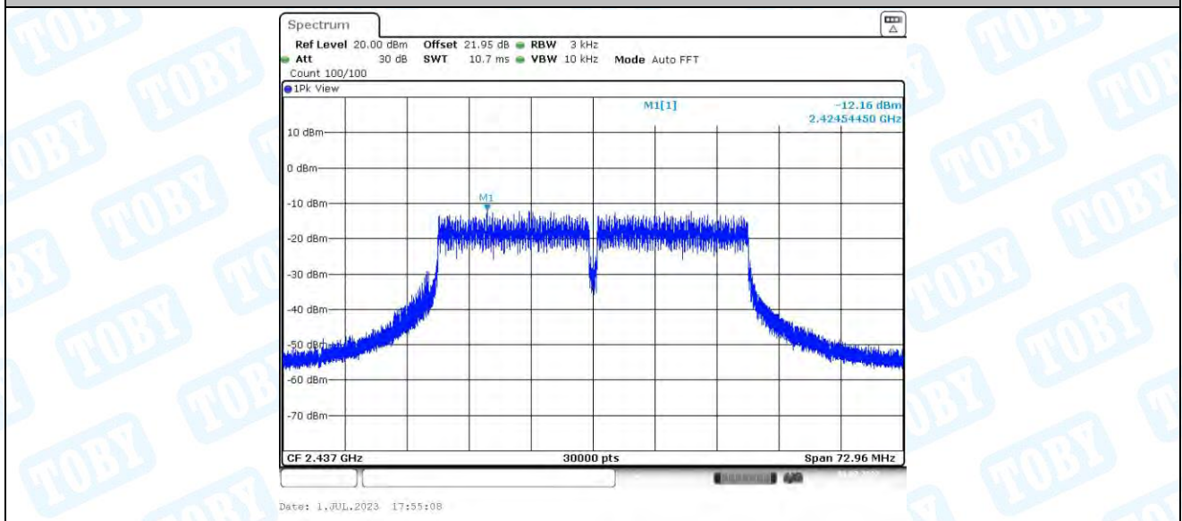
11N40MIMO_Ant3_2437
