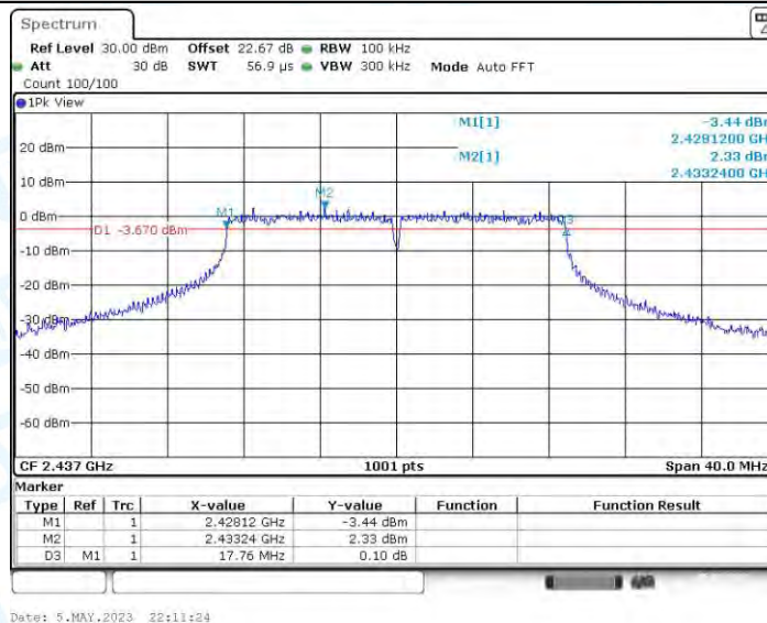
11N20MIMO_Ant3_2437
