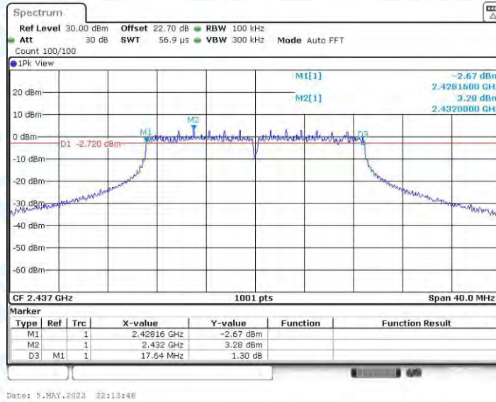
11N20MIMO_Ant4_2437
