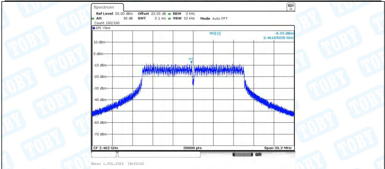
11N20MIMO_Ant3_2462
