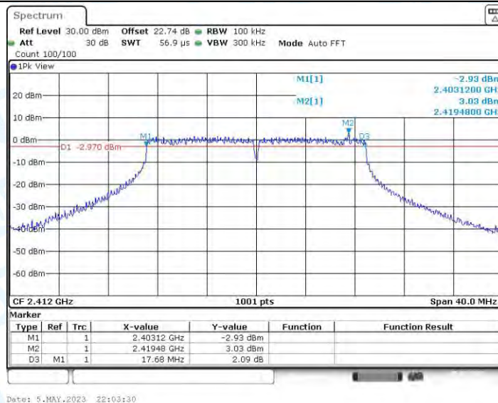
11N20MIMO_Ant4_2412
