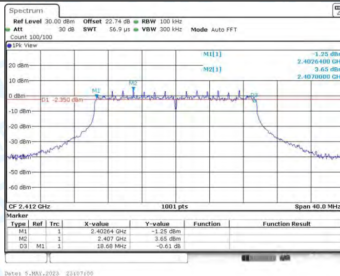
11AX20MIMO_Ant4_2412
