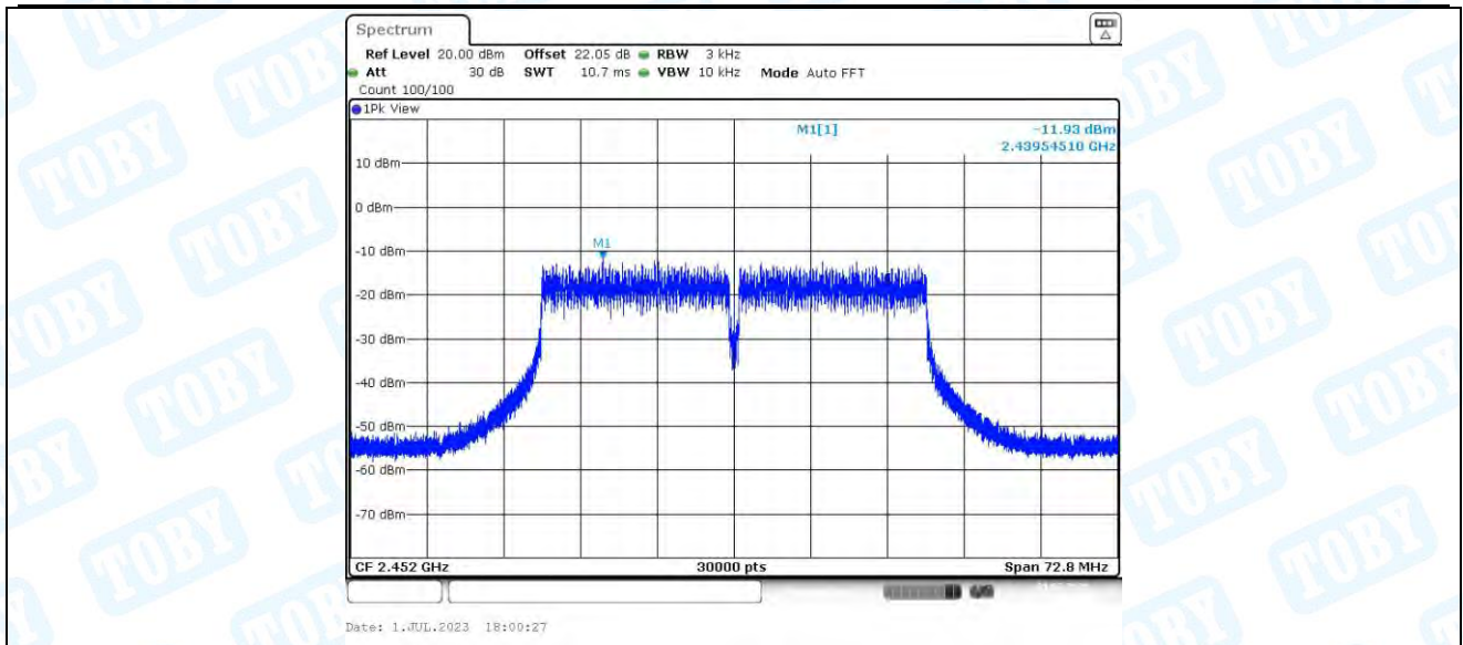
11N40MIMO_Ant3_2452
