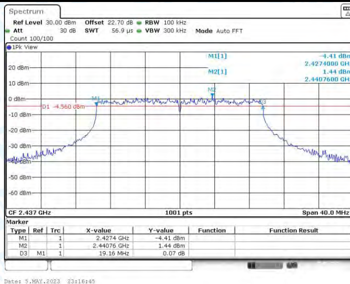
11AX20MIMO_Ant4_2437
