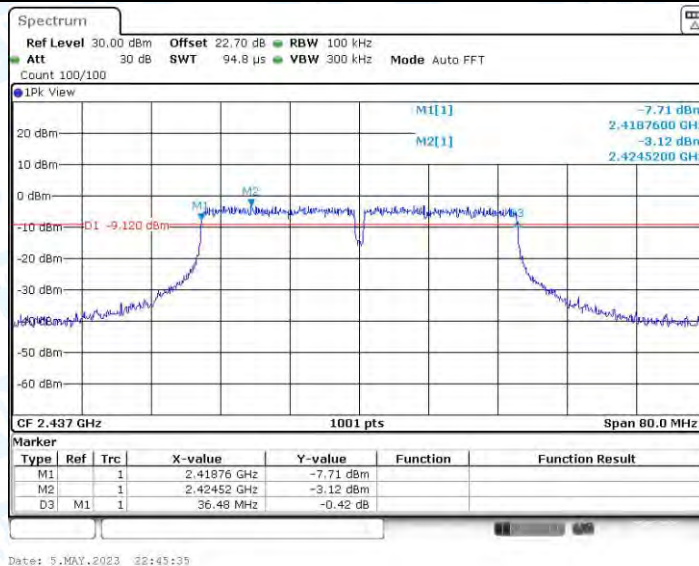
11N40MIMO_Ant4_2437
