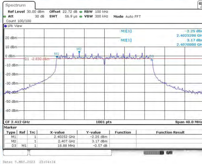
11AX20MIMO_Ant3_2412
