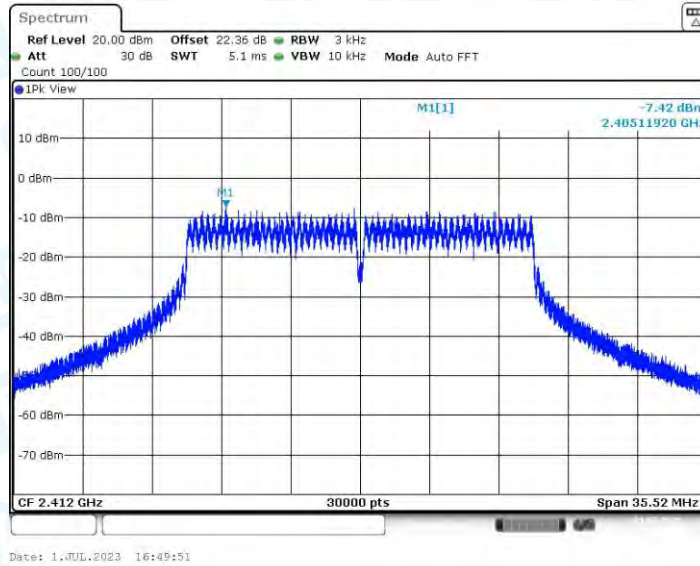
11N20MIMO_Ant3_2412
