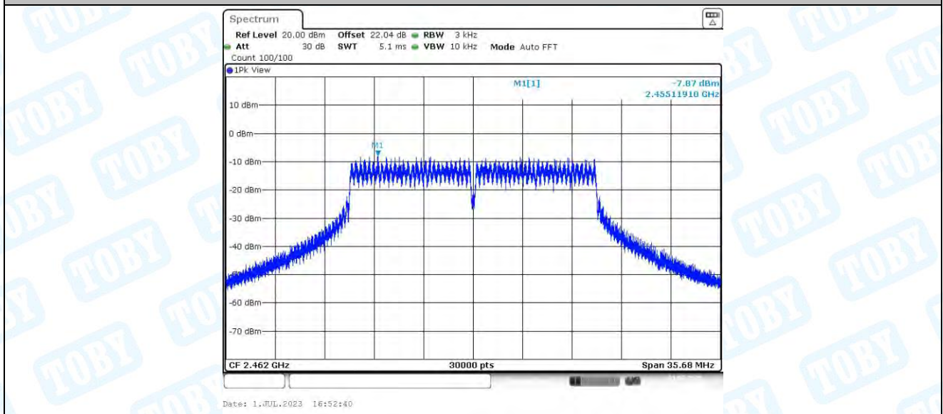
11N20MIMO_Ant4_2462
