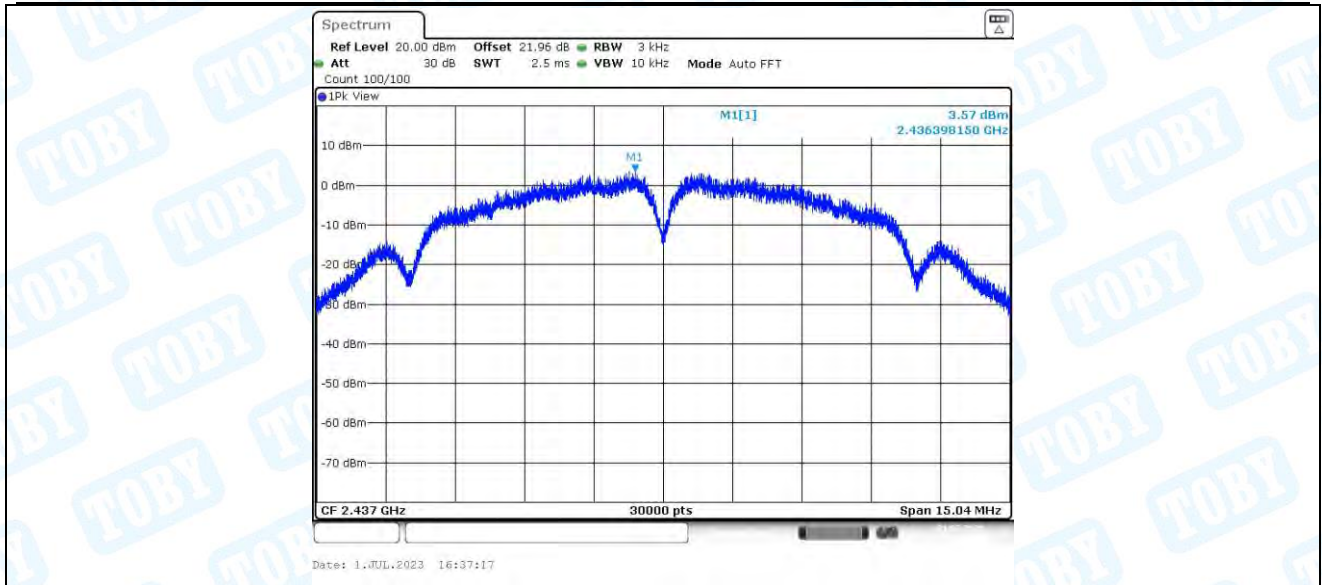
11B_Ant4_2437
