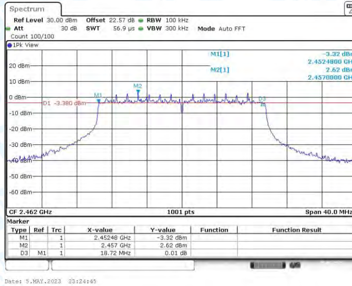
11AX20MIMO_Ant3_2462
