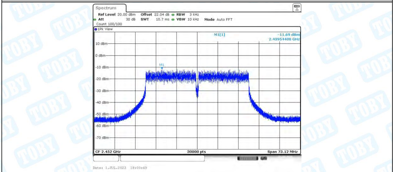
11N40MIMO_Ant4_2452
