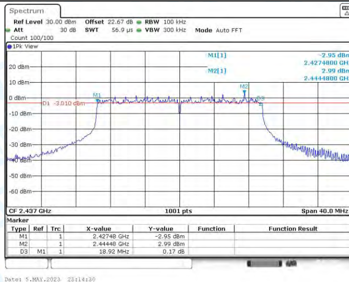
11AX20MIMO_Ant3_2437
