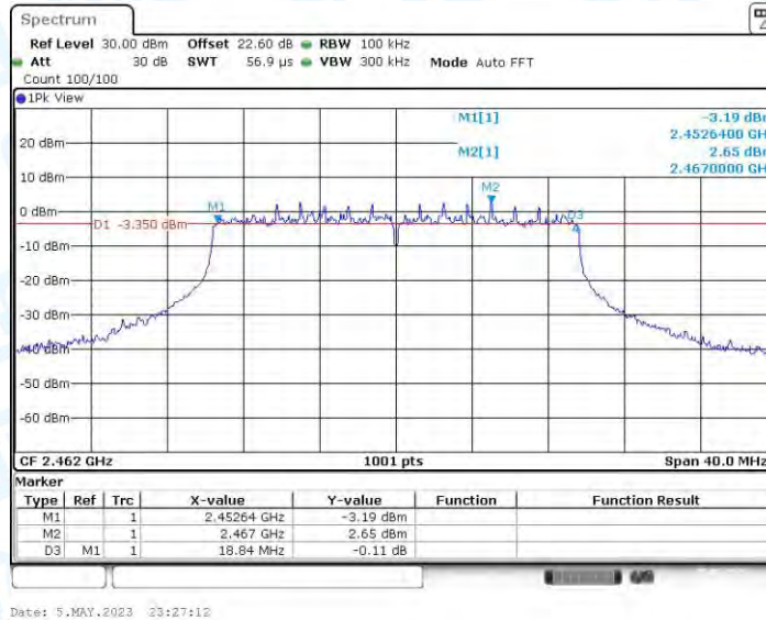
11AX20MIMO_Ant4_2462
