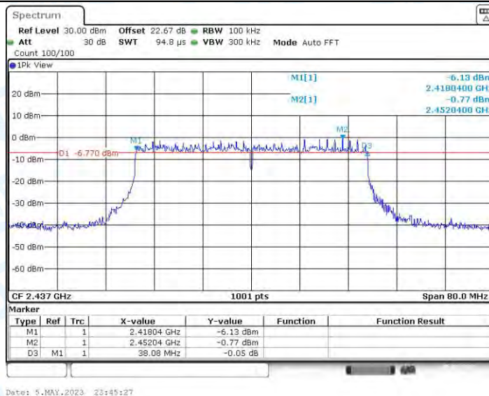
11AX40MIMO_Ant3_2437
