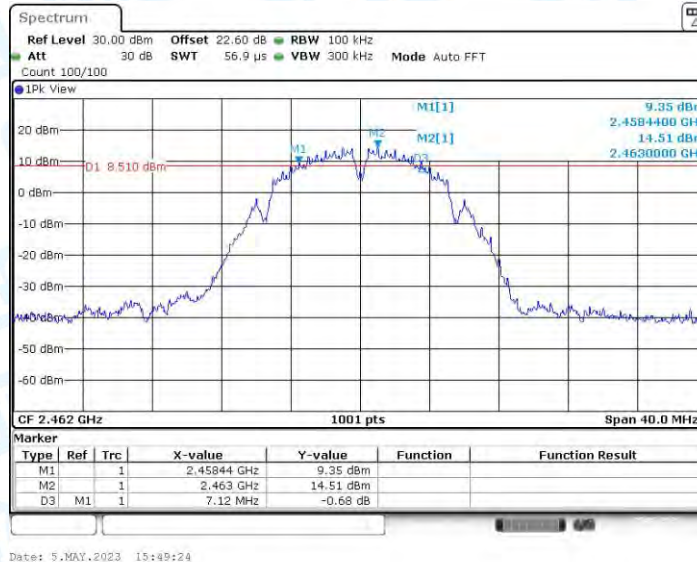
11B_Ant4_2462
