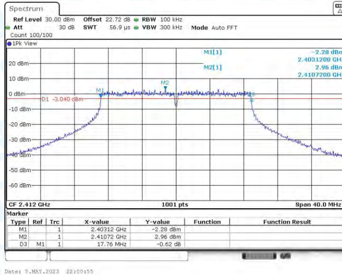
11N20MIMO_Ant3_2412
