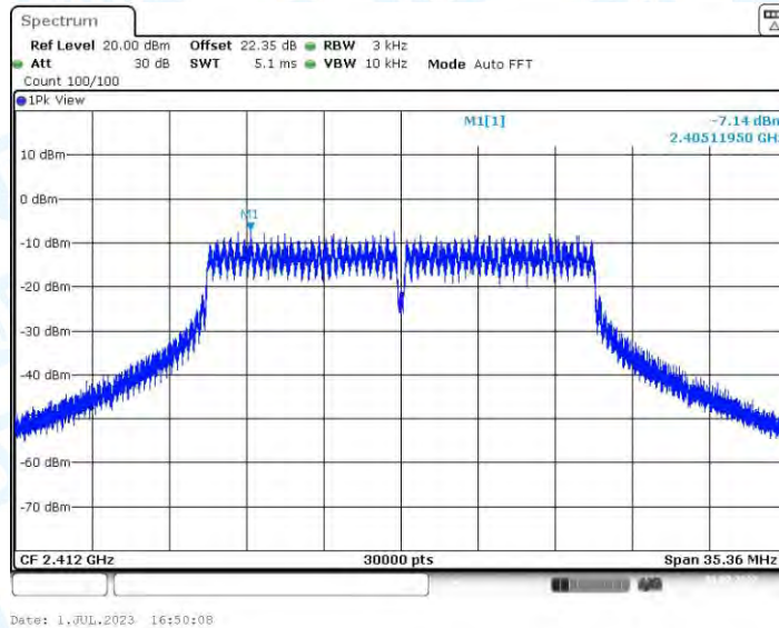
11N20MIMO_Ant4_2412
