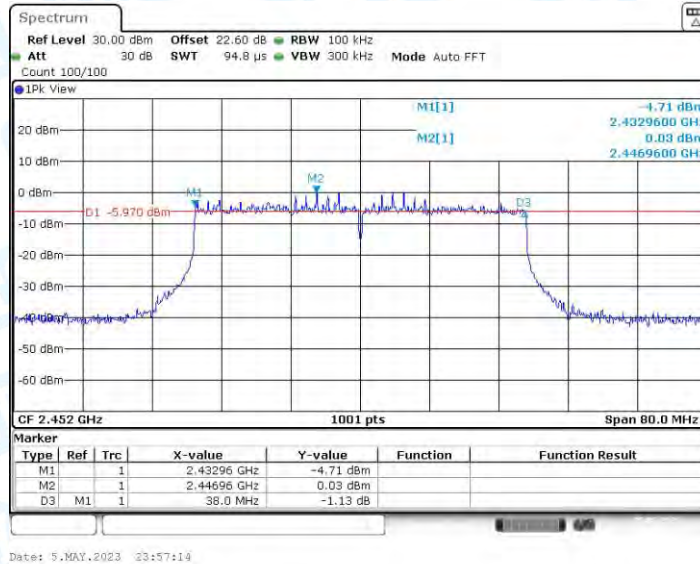
11AX40MIMO_Ant4_2452
