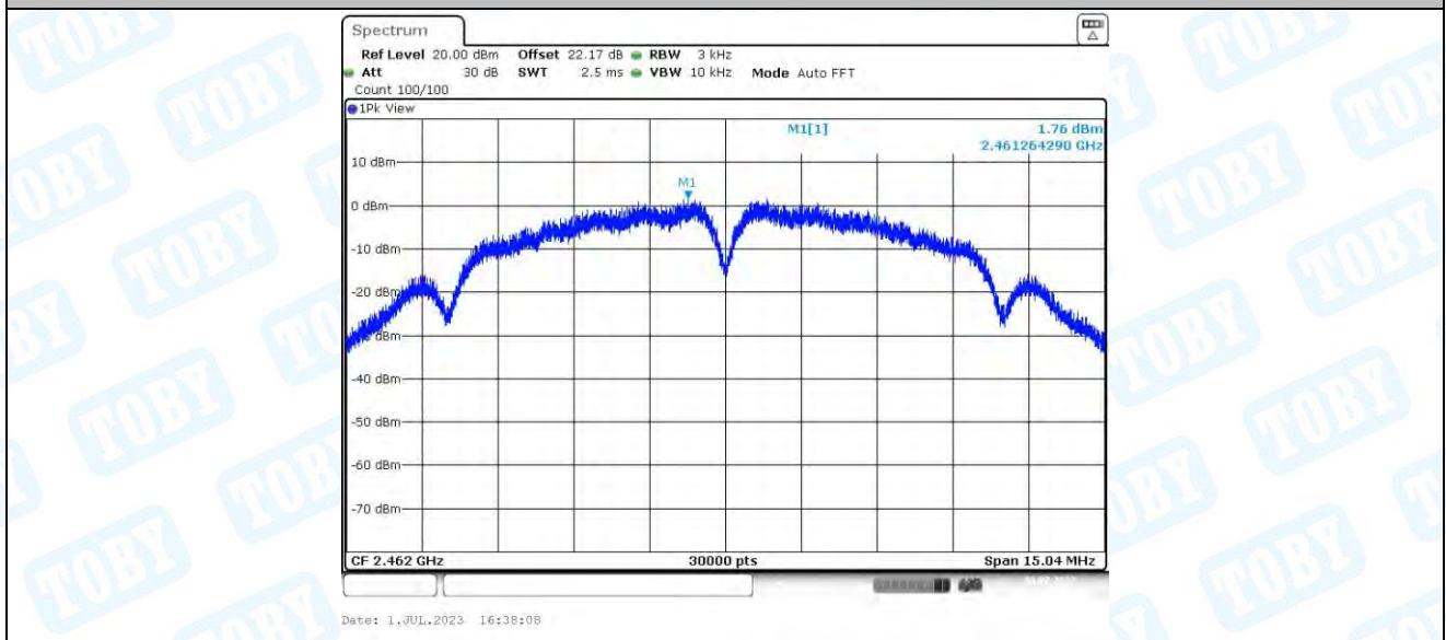
11B_Ant2_2462
