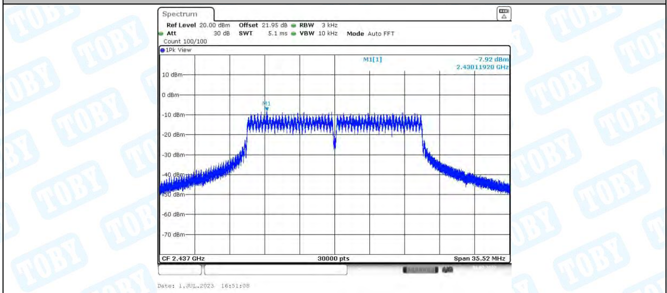
11N20MIMO_Ant3_2437
