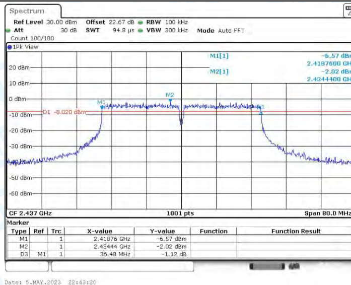
11N40MIMO_Ant3_2437
