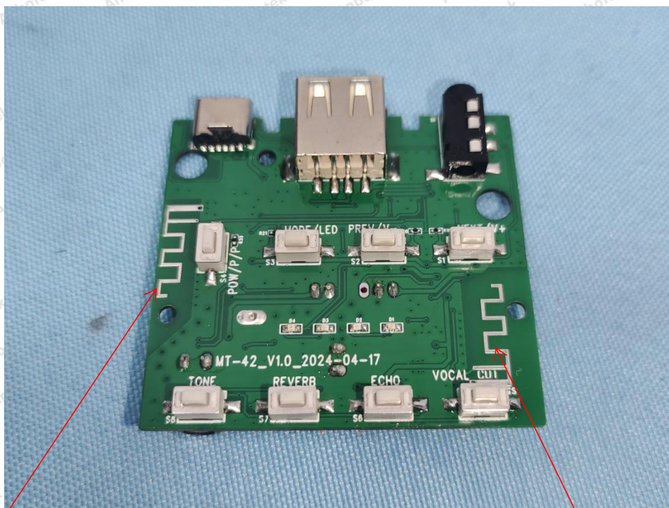
Module 1 ANT
