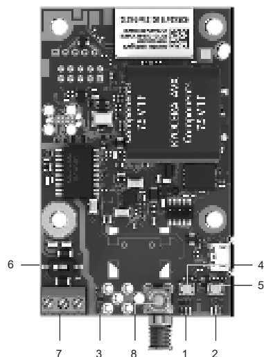
CIM 290 正面図
