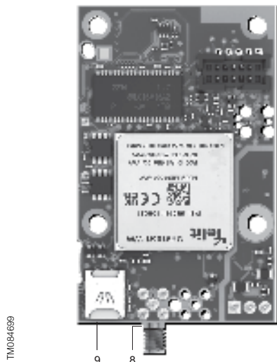
CIM 290 後視圖
