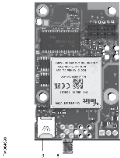
CIM 290, Rückansicht
