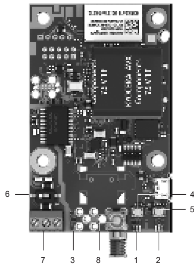
CIM 290, Vorderansicht
