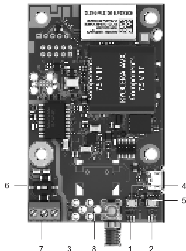
CIM 290 framifrån
