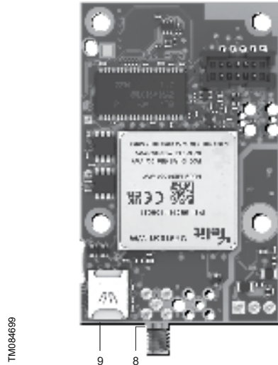
CIM 290 후면
