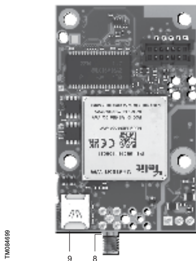
CIM 290 背面図
