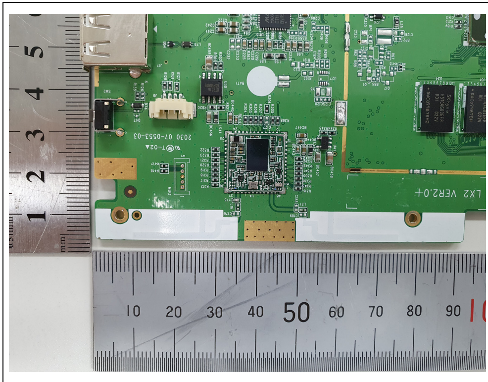
<Antenna _ Front>
