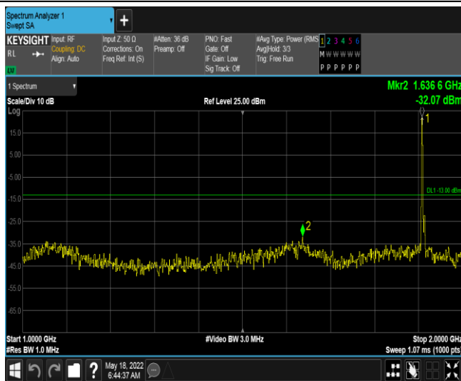
Band2-3MHz-16QAM-19185-1RB#0-Range2:1000~2000MHz
