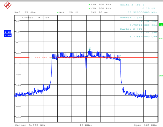
11AC80SISO-Ant1-5775
