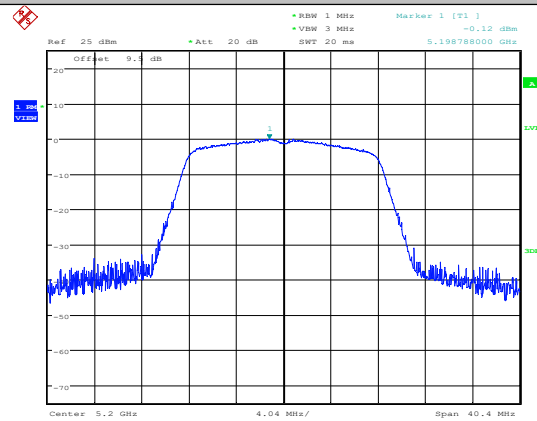
11A-Ant1-5200
