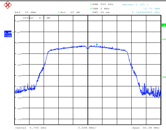
11A-Ant1-5745
