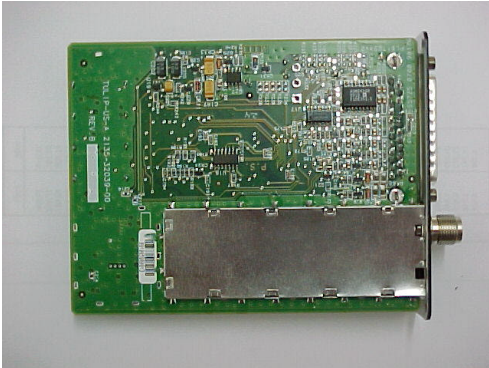
TULIP_US print side
