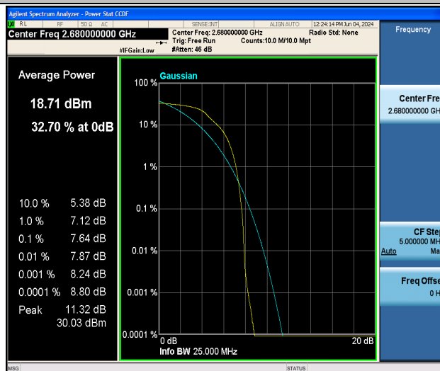
Band41-20MHz-QPSK-41490-1RB#0-PASS
