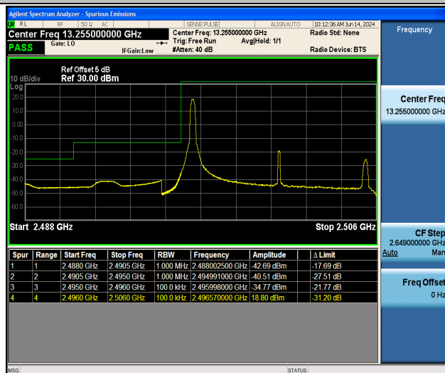
Band41_10MHz_QPSK_39700_1RB#0
