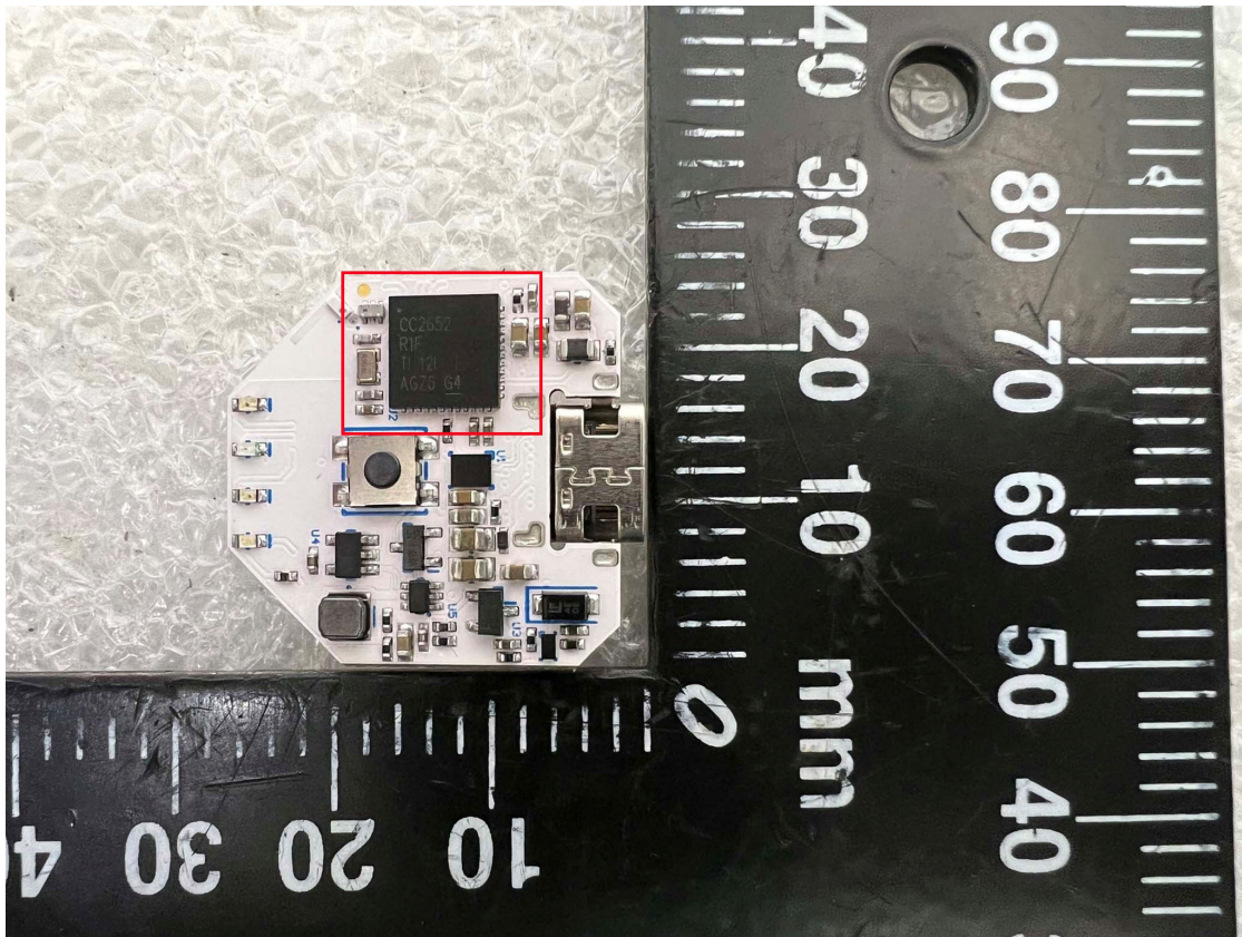
EUT-3. Module CC2652
