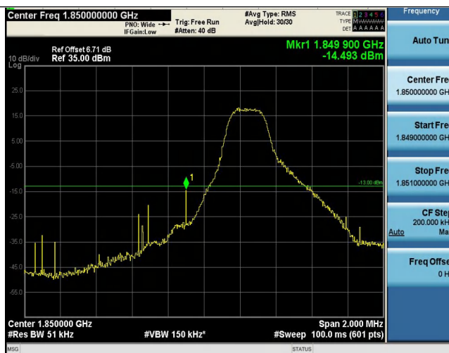
Band2-3MHz-QPSK-18615-1RB#14
