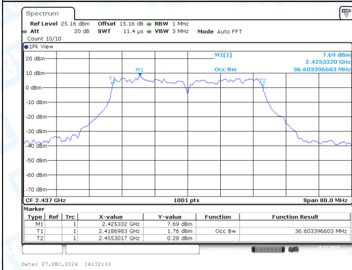
11N40MIMO-Ant1-2437
