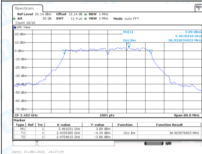
11N40MIMO-Ant1-2452
