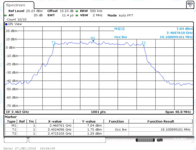
11AX20MIMO-Ant2-2462
