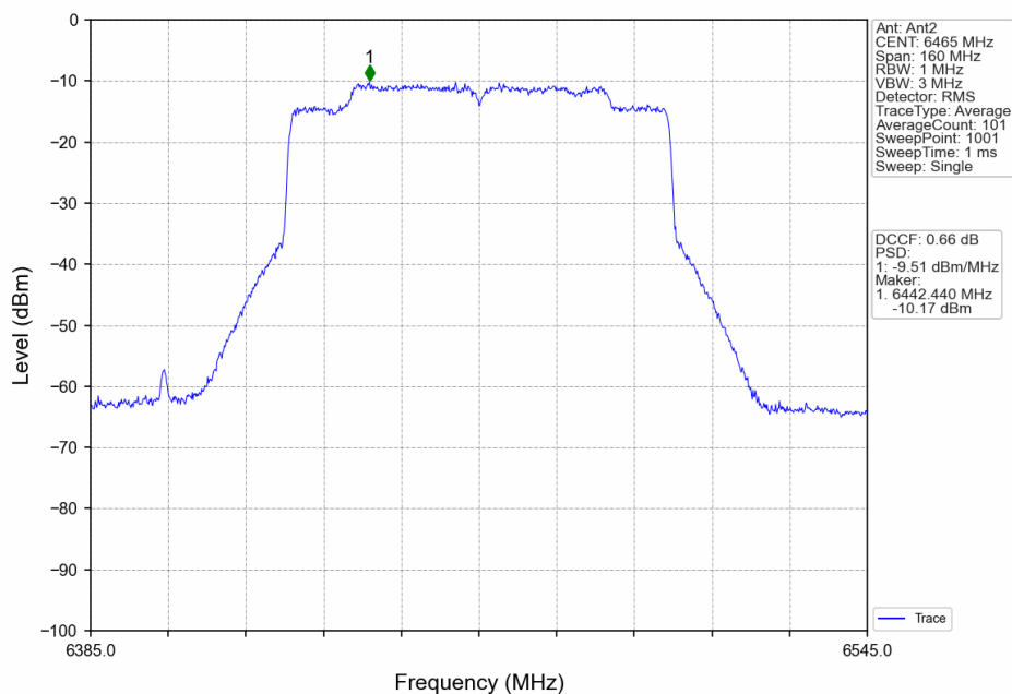
802.11ax(HEW80)_LCH_6465MHz_RU996_Left_MIMO_NTNV
