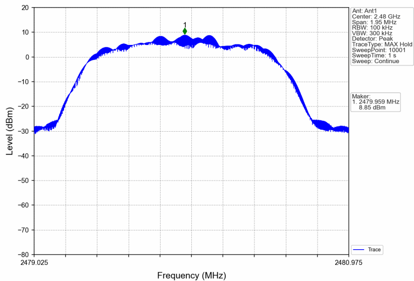
8DPSK 3DH5 HCH 2480MHz Ant1 NTN
