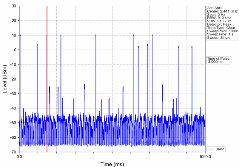
Pi/4DQPSK_2DH5_HOPP_Ant1_NTNV
