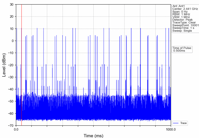
Pi/4DQPSK_2DH3_HOPP_Ant1_NTNV
