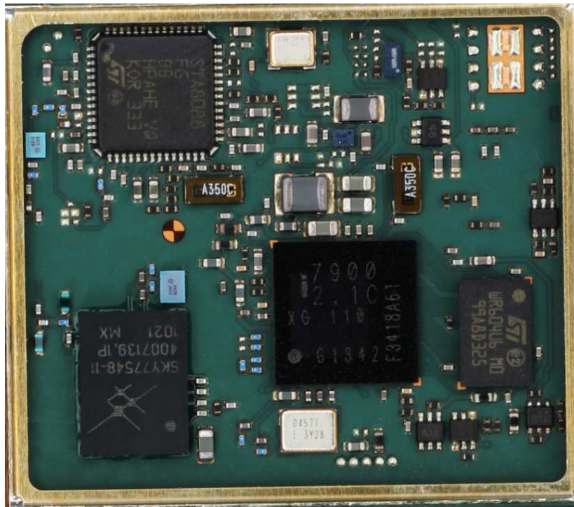
AGS2-E Top side
