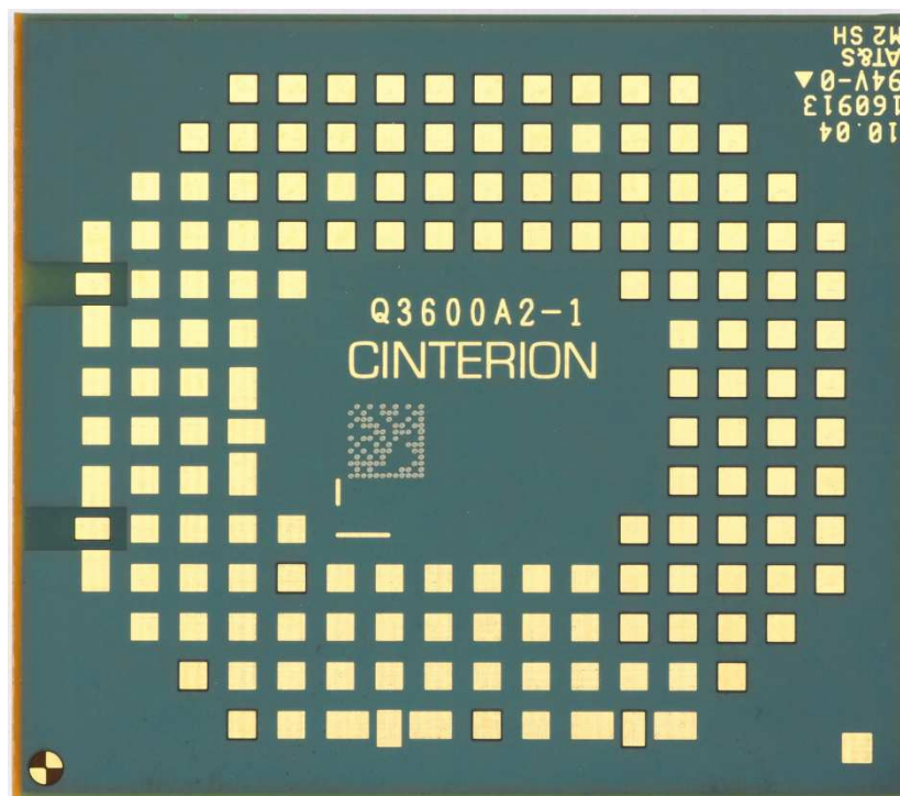
AGS2-E Bottom Side
