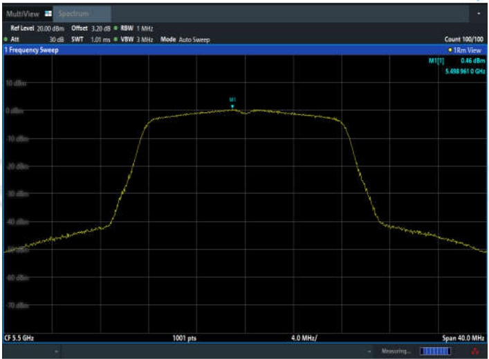
11A_Ant2_5500
