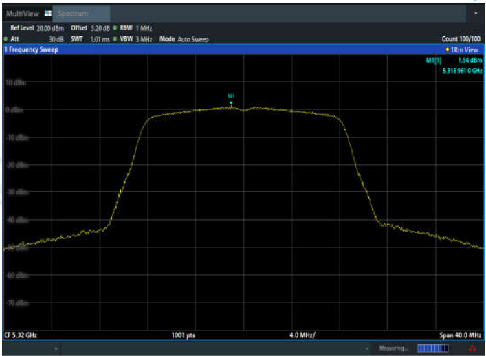
11A_Ant2_5320
