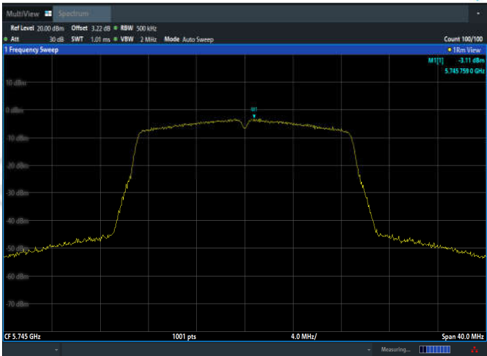
11N20SISO_Ant2_5745
