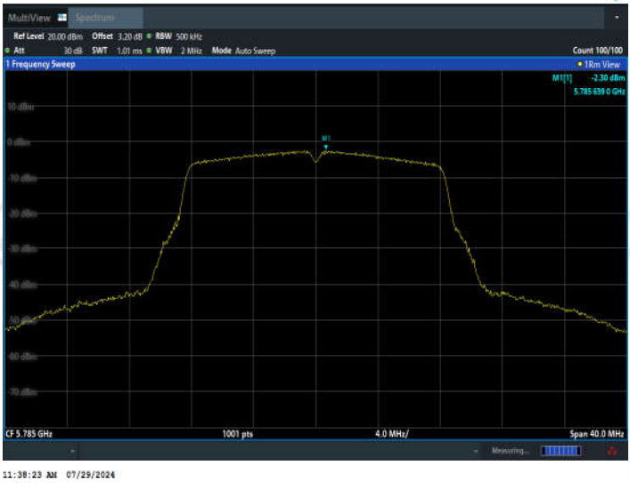
11A_Ant2_5785
