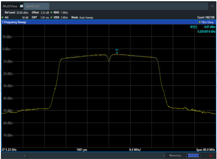
11N40SISO_Ant2_5230
