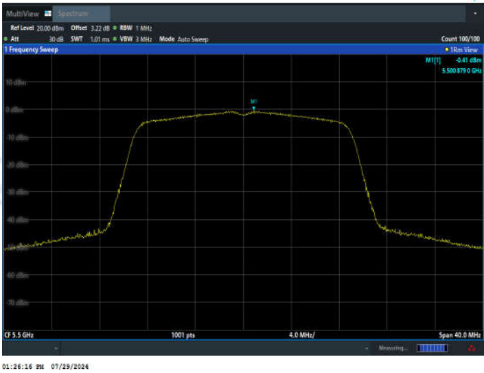
11N20SISO_Ant2_5500
