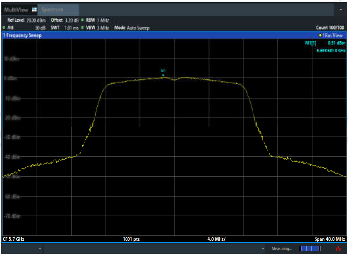
11A_Ant2_5700
