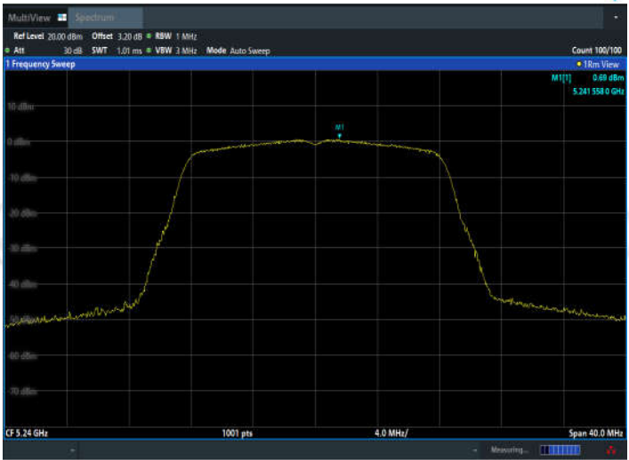
11A_Ant2_5240
