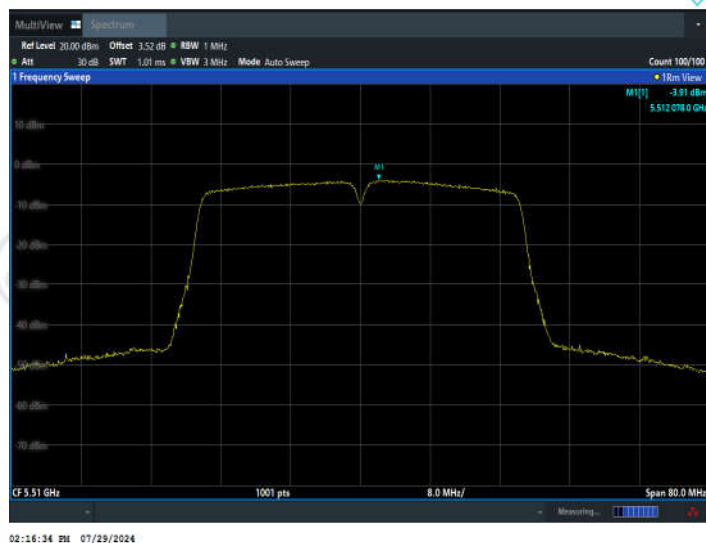
11N40SISO_Ant2_5510
