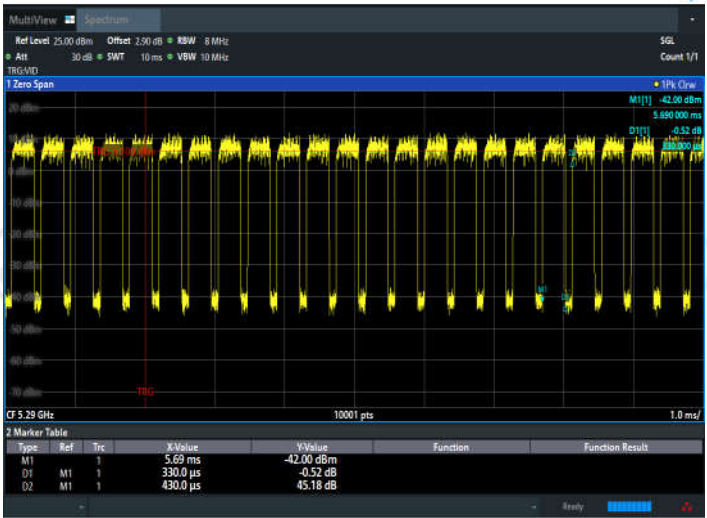
11AC80SISO_Ant2_5290
