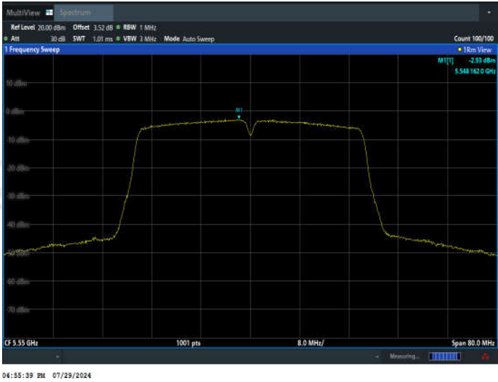
11AC40SISO_Ant2_5550
