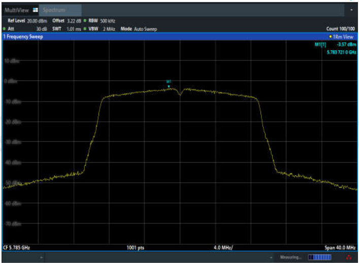
11N20SISO_Ant2_5785
