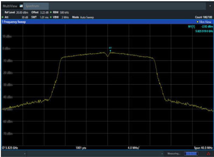
11N20SISO_Ant2_5825
