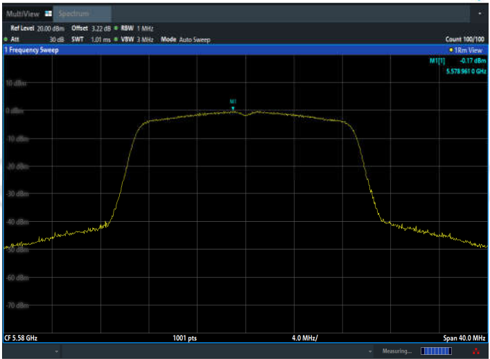
11N20SISO_Ant2_5580
