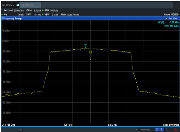
11N40SISO_Ant2_5755
