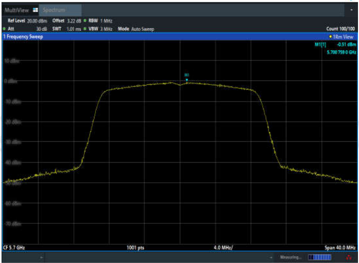
11N20SISO_Ant2_5700
