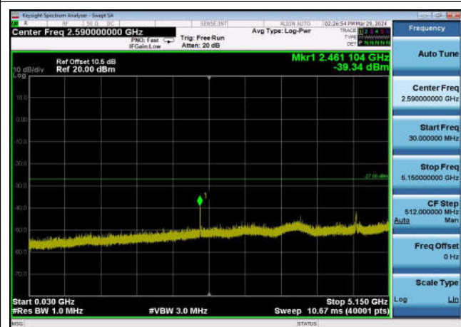
U-NII-2a ,Plot 2,30MHz~5150MHz-802.11 ac(20MHz),5300MHz,Ant1
