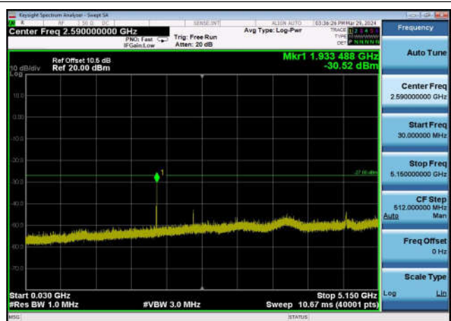
U-NII-2a ,Plot 2,30MHz~5150MHz-802.11 ac(20MHz),5320MHz,Ant1
