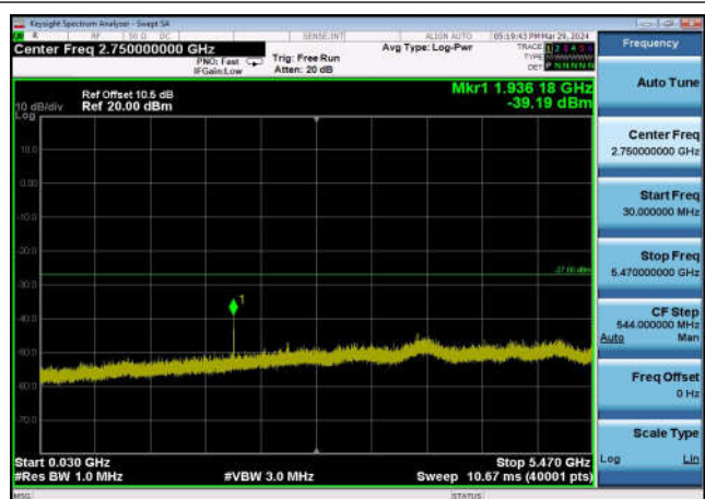
U-NII-2c ,Plot 2,30MHz~5470MHz-802.11 ac(20MHz),5700MHz,Ant1
