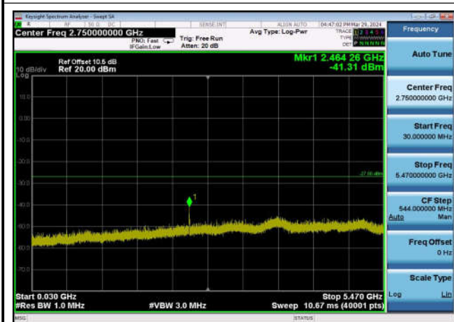
U-NII-2c ,Plot 2,30MHz~5470MHz-802.11 n(20MHz),5580MHz,Ant1
