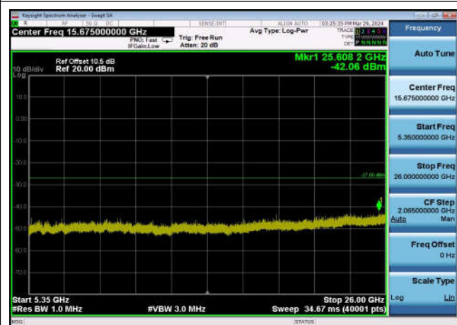
U-NII-2a ,Plot 3,5350MHz~26000MHz-802 .11ac(20MHz),5320MHz,Ant1
