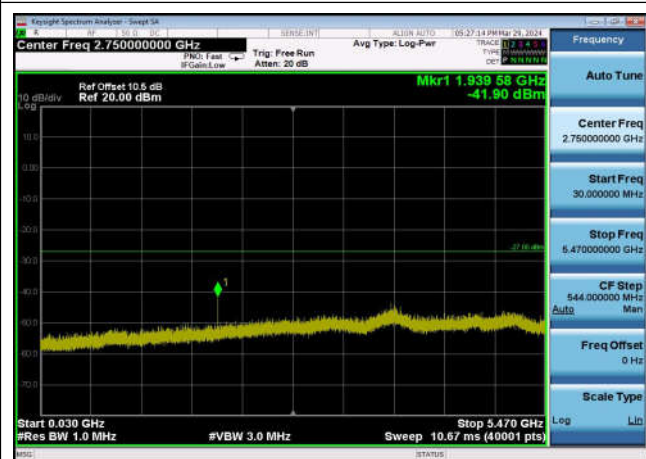
U-NII-2c ,Plot 2,30MHz~5470MHz-802.11 ac(40MHz),5510MHz,Ant1
