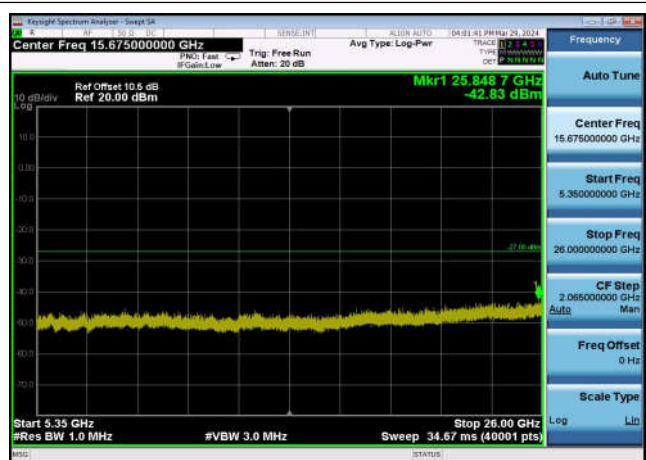
U-NII-2a ,Plot 3,5350MHz~26000MHz-802 .11ac(80MHz),5290MHz,Ant1
