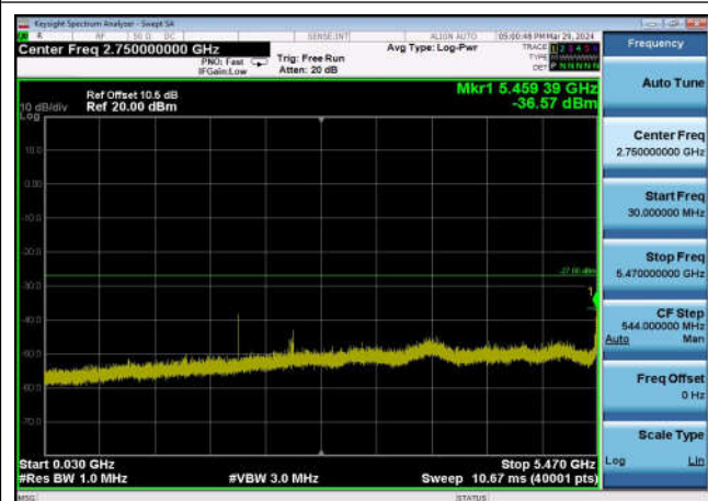
U-NII-2c ,Plot 2,30MHz~5470MHz-802.11 n(40MHz),5670MHz,Ant1
