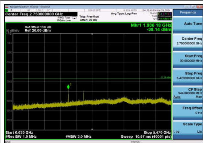
U-NII-2c ,Plot 2,30MHz~5470MHz-802.11 ac(20MHz),5580MHz,Ant1
