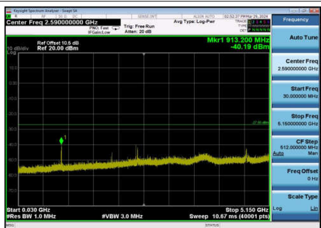
U-NII-2a ,Plot 2,30MHz~5150MHz-802.11 n(20MHz),5320MHz,Ant1
