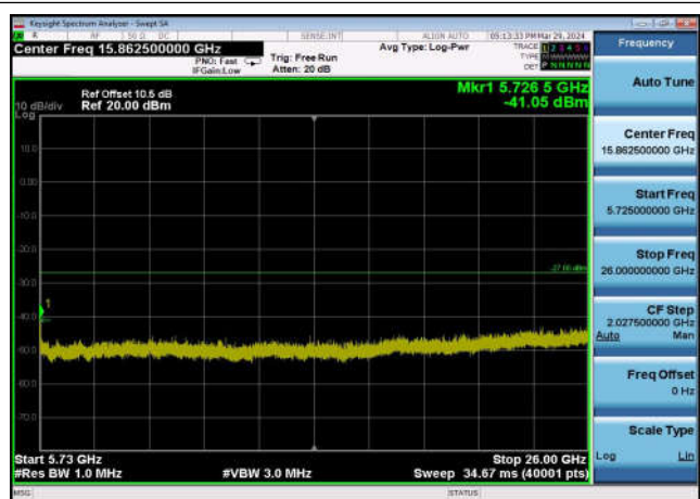
U-NII-2c ,Plot 3,5725MHz~26000MHz-802.11n(40MHz),5670MHz,Ant1
