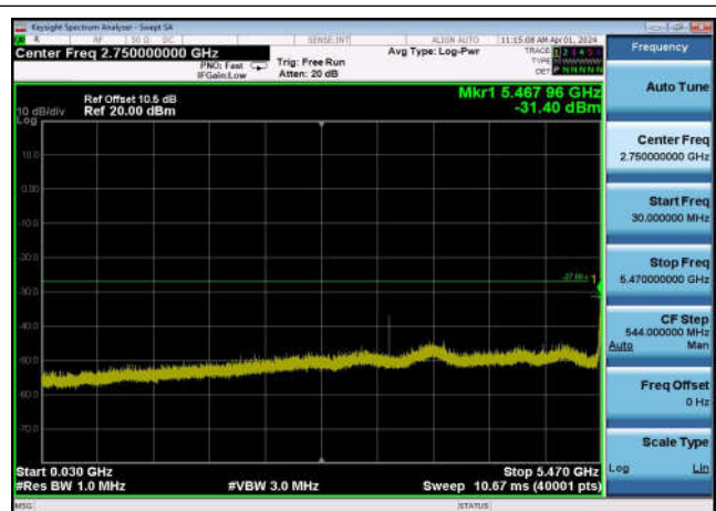
U-NII-2c ,Plot 2,30MHz~5470MHz-802.11 n(20MHz),5700MHz,Ant1
