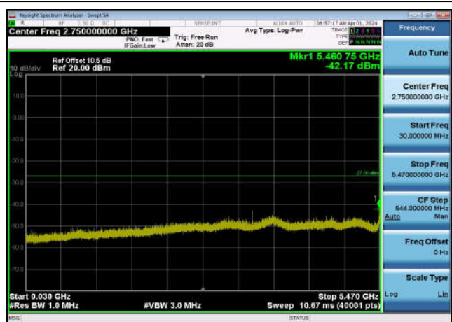
U-NII-2c ,Plot 2,30MHz~5470MHz-802.11 ac(40MHz),5550MHz,Ant1
