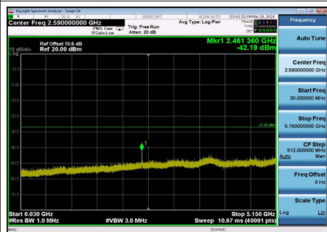
U-NII-2a ,Plot 2,30MHz~5150MHz-802.11 ac(80MHz),5290MHz,Ant1
