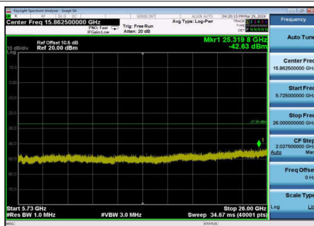
U-NII-2c ,Plot 3,5725MHz~26000MHz-802.11ac(20MHz),5500MHz,Ant1
