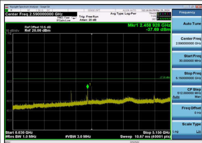
U-NII-2a ,Plot 2,30MHz~5150MHz-802.11 a(20MHz),5320MHz,Ant1
