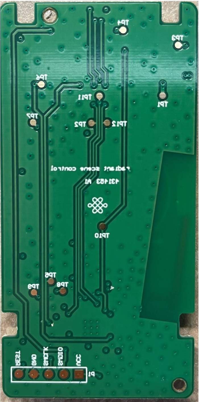
PCBA - BOT
