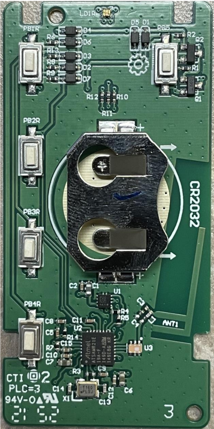
PCBA - TOP
